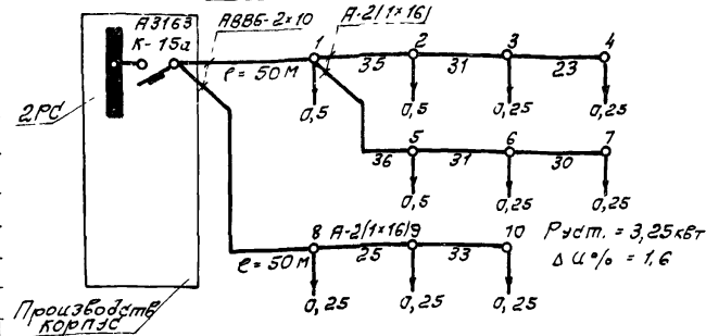
Расчетная схема осветительной сети ~ 380/220В
