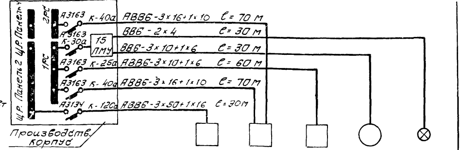
Расчетная схема силовой сети ~ 380/220В
