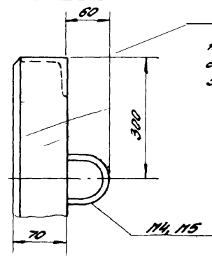
Деталь, Б''
