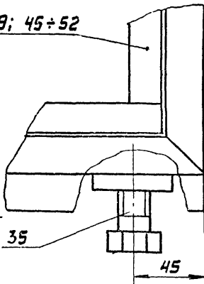
Г-Г лист 2 M 1:1
