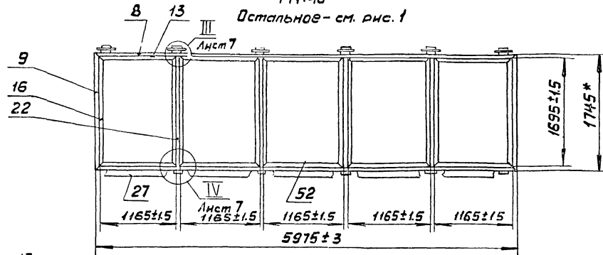
Рис 13 М 1:40
