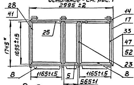
Рис. 9 М1:40 Остальное - см. рис. 1
