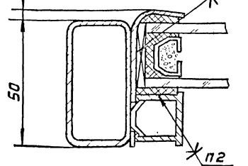
Г-Г лист M1:1
