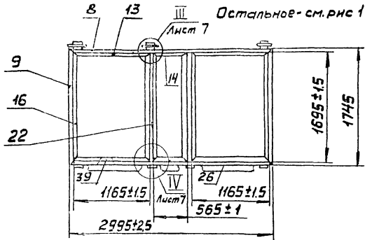
Рис.12 М 1:40
