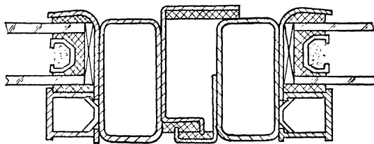
Д-Д M1:1
