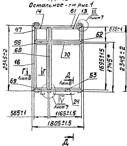
Рис.12 М 1:40
