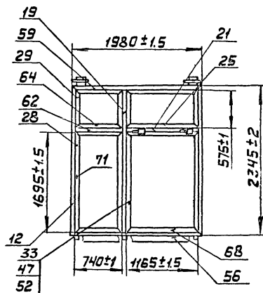
Рис. 15 М 1:40 Остальное - см. рис. 1
