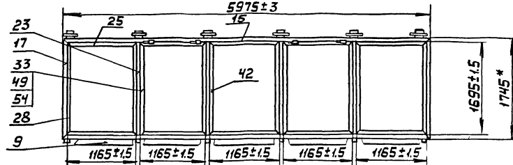
Рис. 10 М1:40 Остальное - см. рис. 1
