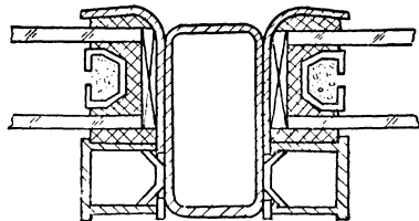
Д-Д M1:1
