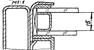
Б-Б M1:1
