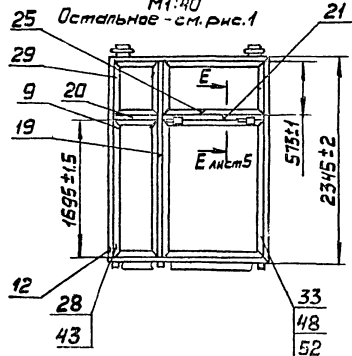
Рис. 9 М1:40 Остальное - см. рис. 1
