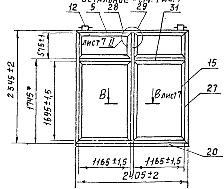
Рис. 13 М 1:40
