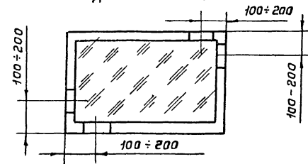
Подвеска боковая
