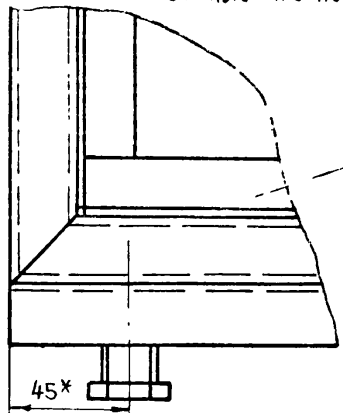
II ЛИСТ 1 М 1:2 ШТАПИК И ОТФКЛУ НЕ ПОКАЗАНЫ
