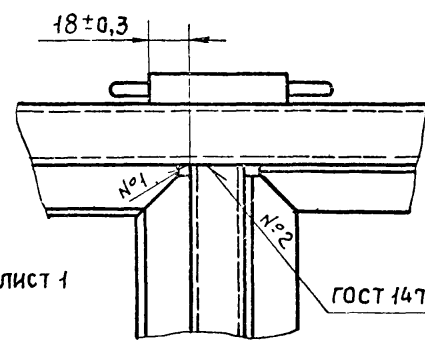
III- III ЛИСТ 1,2,3,4,5,6 М 1:2
