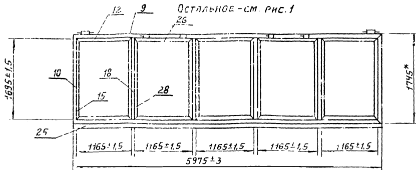
Рис 10 М 1:40
