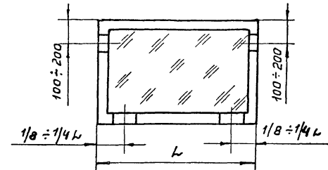
Подвеска боковая
