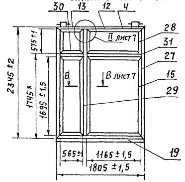
Рис. 12 М 1:40
