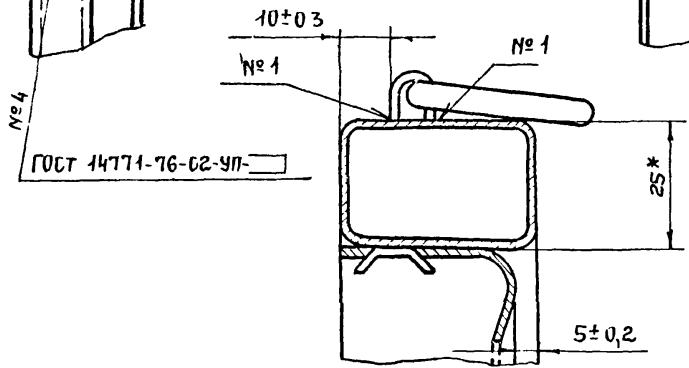
ГОСТ 14771-76-С2-УП
