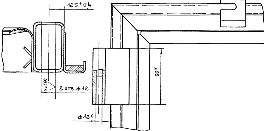
Ж - Ж лист 1 М 1:1
