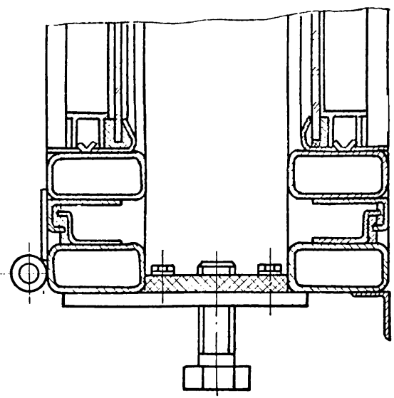
Б-Б ЛИСТ 1 М 1:2
