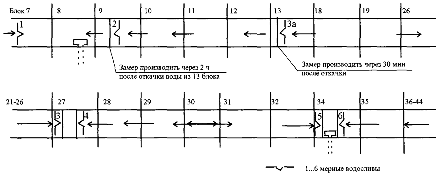
Схема размещения КИА на ГЭС Раякоски. ГЭС-6. Водосливы
