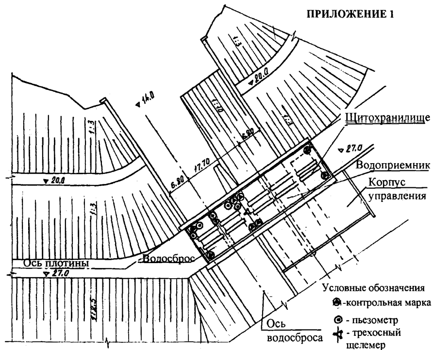
Схема размещения КИА на бетонных сооружениях Нижне-Териберского гидроузла
