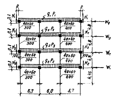
Схема поперечной рамы и ее загрузки в знаменателе под размерами сечений колонн указана марка бетона
