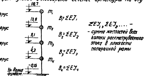
Динам. расчетная схема каркаса здания в поперечном направлении
