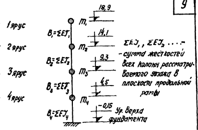
Динамическая расчетная схема каркаса здания в продольном направлении
