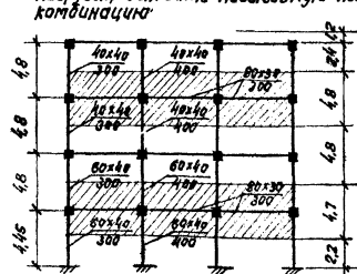
Схема распределения ярусных масс в поперечных рамах
