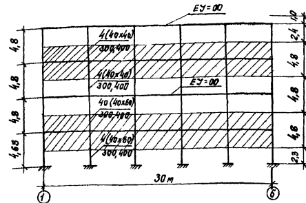
Схема распределения ярусных масс в продольных рамах
