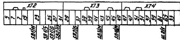
ПОД. 8 КНОПКА РЕ ДИ НСП.3 SB1
