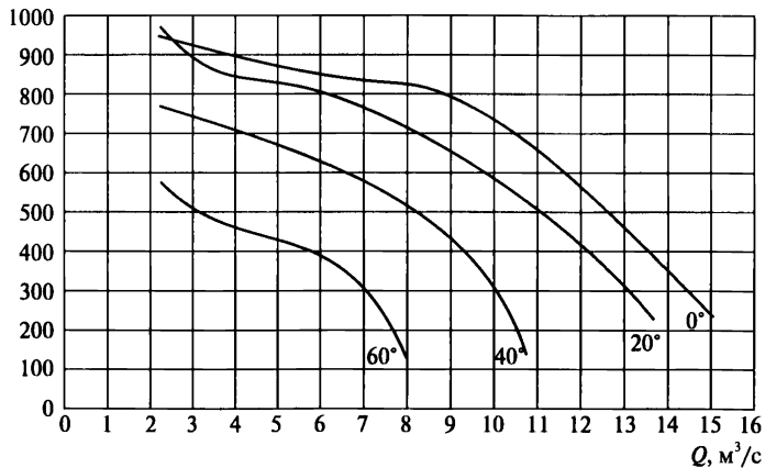
Рис. 12.1. Аэродинамическая характеристика вентилятора ВЦГ-7М
