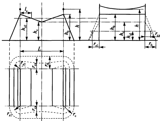
Рис. 14.7. Зона защиты двойного тросового молниеотвода
