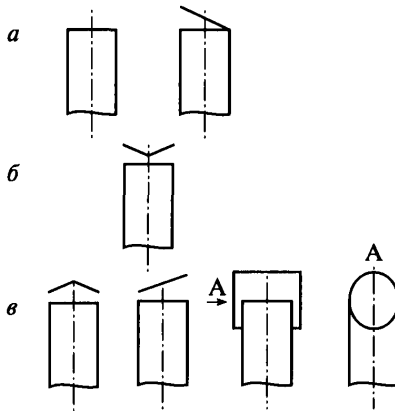
Рис. 14.2. Конструкции колпаков
