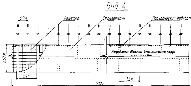
Рис. 8.1. Принципиальная схема сооружения смесительной камеры
