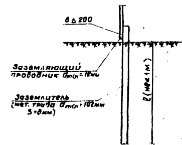
Пример устройства заземлителей у опор на склоне
