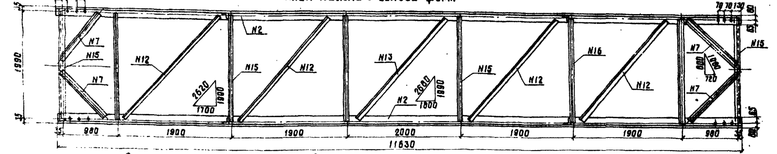
Конструкция хребта по краештвину для обслуживания ЛЭП
