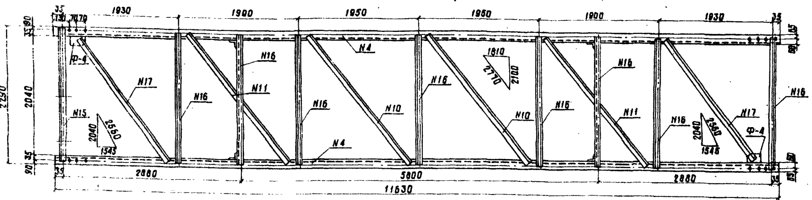
План нижних связей ферм
