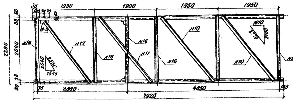
План нижних связей ферм
