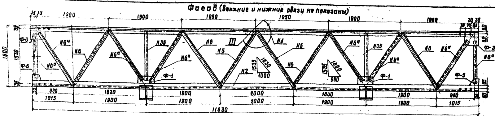
План верхних связей ферм
