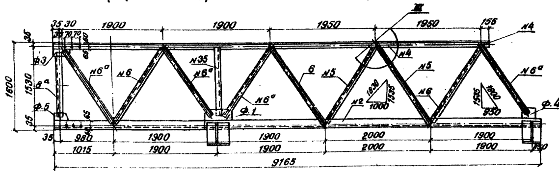
План верхних связей ферм
