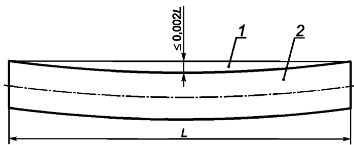
1 — натянутая струна или проволока; 2 — труба
