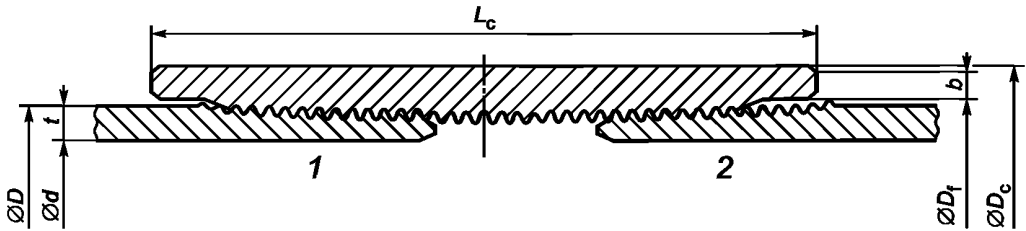
1 — основное механическое свинчивание; 2 — ручное свинчивание; L_c — заданная минимальная длина муфты; D_c — заданный наружный диаметр муфты; D_t — заданный диаметр фаски в плоскости торца муфты; b — заданная ширина упорного торца; D — наружный диаметр трубы; t — толщина стенки трубы; d — внутренний диаметр трубы
