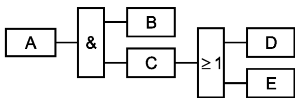
Рисунок 5 — Представление вентиляей и событий в виде прямоугольников
