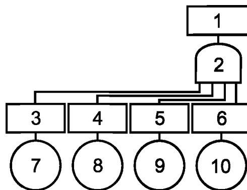
Рисунок 3 — Представление параллельной системы в виде ДН
