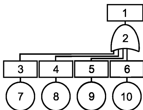
Рисунок 2 — Представление последовательной системы в виде ДН
