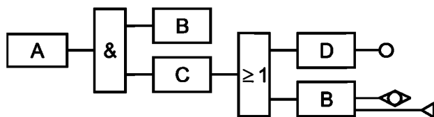
Рисунок 7 — Пример событий, вызванных общими причинами и изображенных в виде прямоугольных вентилей
