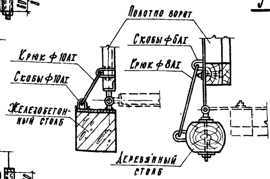
ДЕТАЛИ ФИКСАЦИИ СТВОРОК В ОТКРЫТОМ ПОЛОЖЕНИИ
