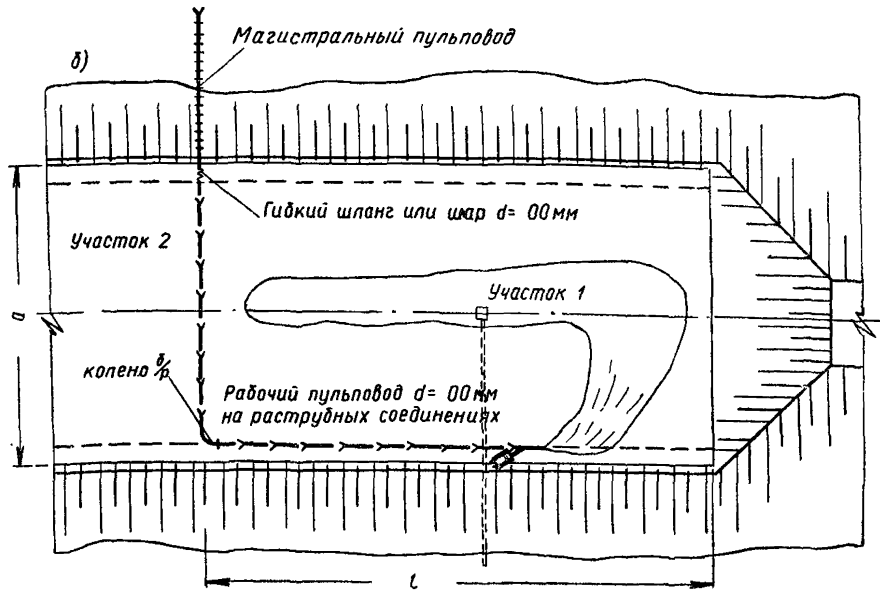
Рис. 3 Схемы организации намыва а — с переключателем пульпы; б — без переключателя пульпы
