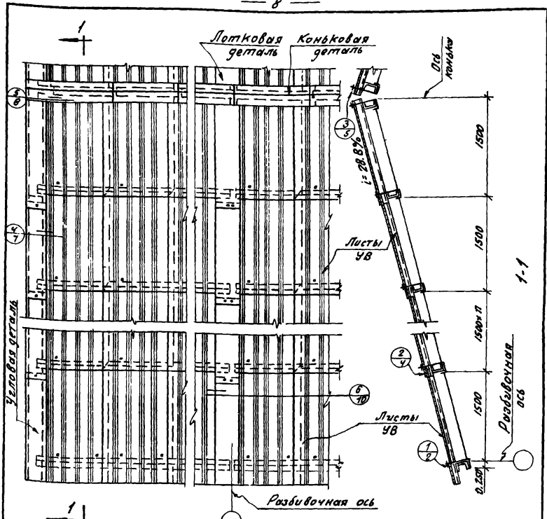
Маркировочный план покрытия.
