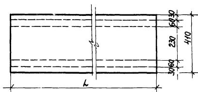
ЛС-2 (для листов ВУ)
