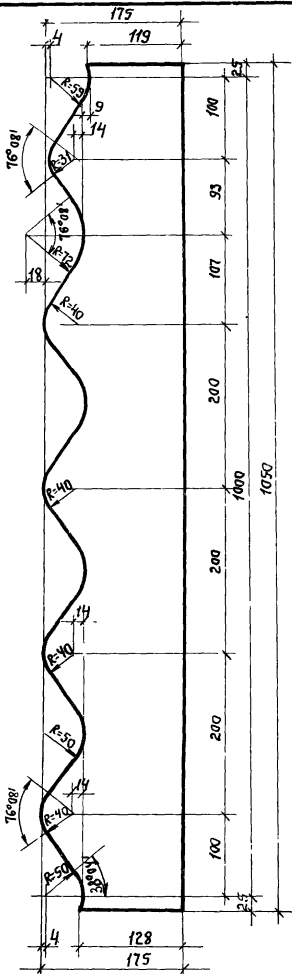
Гребенка ГС-1 (для листов УВ)
