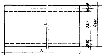
ЛС-1 (для листов УВ)
