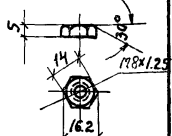
Гайка Г (ГОСТ 5916-62)
