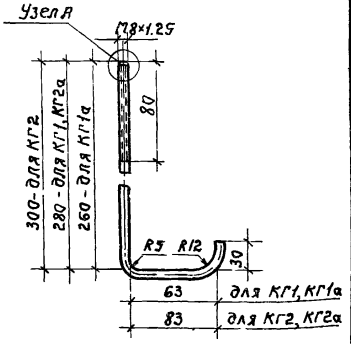
Крюки KГ1, KГ2, KГ1a, KГ2a (для крепления к ступицам швеллерам С160x60x4и С180x80x4)
