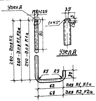
Крюки K1, K2, K1a, K2a (для крепления к прокатным швеллерам С14, 16)
