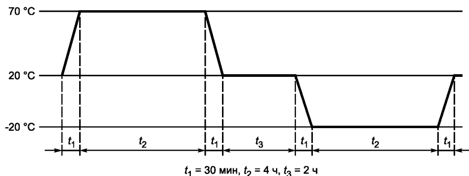
Рисунок 2 — Температурный цикл
