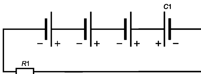
Рисунок 5 — Схема соединений для испытаний на переразряд
