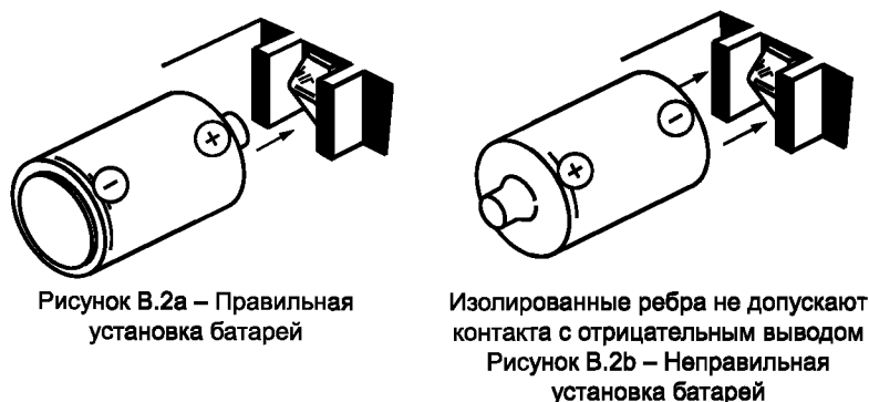
Рисунок В.2 — Положительный контакт, утопленный между ребрами
