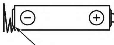
Рисунок В.10а – Пружина проскальзывает снизу оболочки – возможен контакт с металлом
