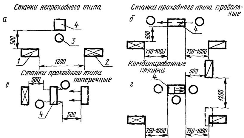
1 — складочное место заготовок; 2 — складочное место деталей; 3 — станочники; 4 — станки Черт. 2
