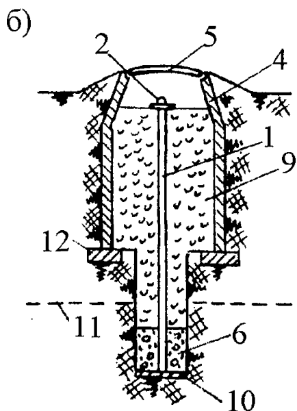
Рис.П.7. Конструкции рабочих реперов для мягких грунтов: а – трубчатый репер; б – репер в котловане; 1 – реперная труба; 2 – реперная головка; 3 – перфорация; 4 – защитный колодец; 5 – крышка колодца; 6 – якорь репера; 7 – защитная труба; 8 – защитная крышка; 9 – теплоизоляционный материал; 10 – анкерная плита; 11 – максимальная глубина промерзания; 12 – основание колодца
