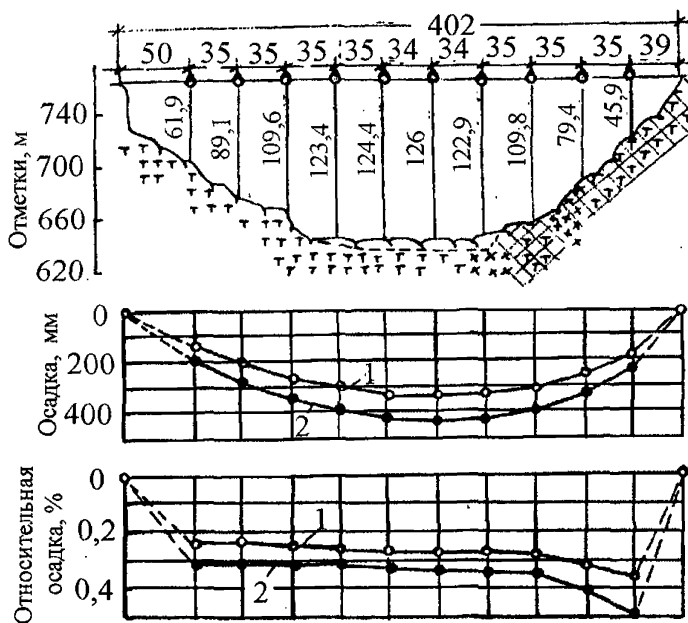
Рис.6.5. Эпюры абсолютной и относительной осадок гребня грунтовой плотины:
