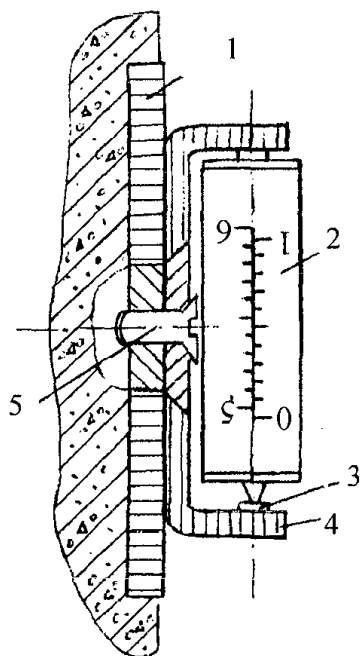
Рис.П.16. Стенная марка конструкции Пискунова:
