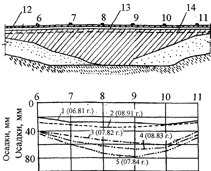
Рис.6.4. Эпюры осадки гребня грунтовой плотины:
