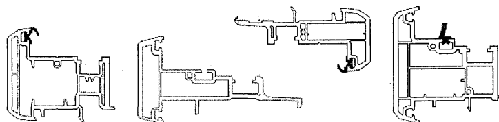
Сечения профилей штульпов
