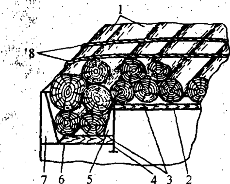
Рис. 8.5.2. Укладка и крепление кряжей на верхней палубе:
