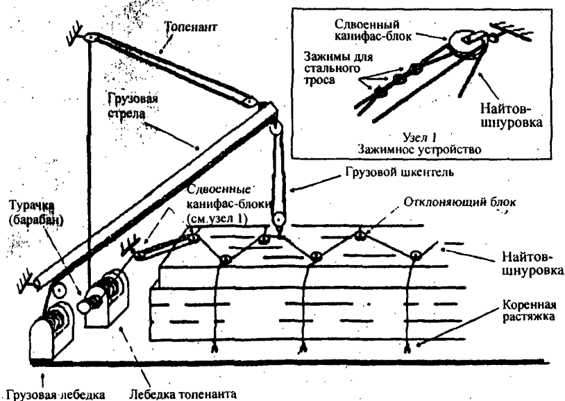
Рис. 8.4.1. Схема обжата каравана методом «шнуровки».
