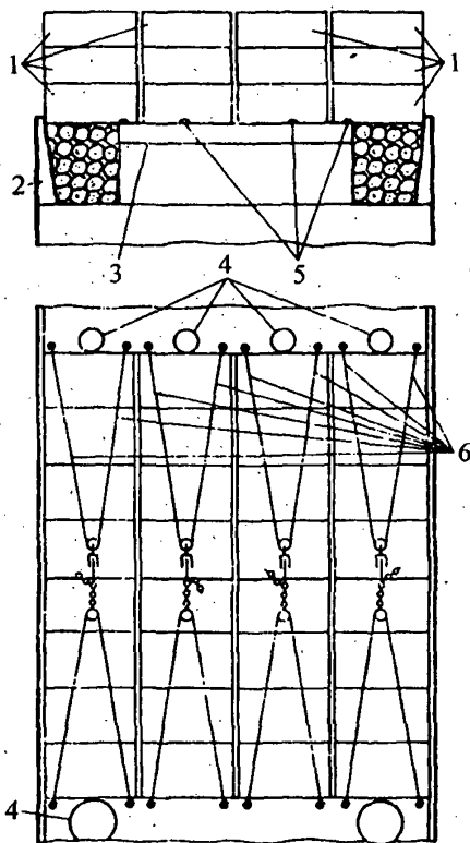
Рис. 8.6.1. Укладка и крепление без стензелей пакетов круглого леса на верхней палубе:
