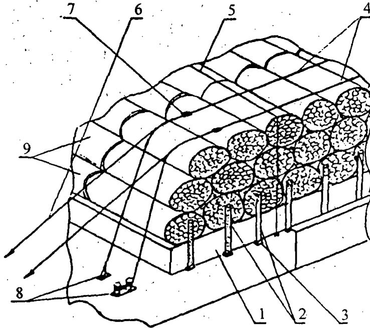
Рис. 8.6.2. Схема укладки и крепления длиномерного круглого леса в пакетах на крышках люков:
