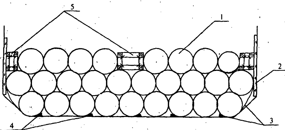
Рис. 7.3. Крепление рулонов, уложенных горизонтально:
