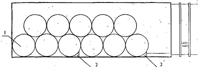
Рис. 6.2. Размещение рулонов в контейнере при укладке на образующую:
