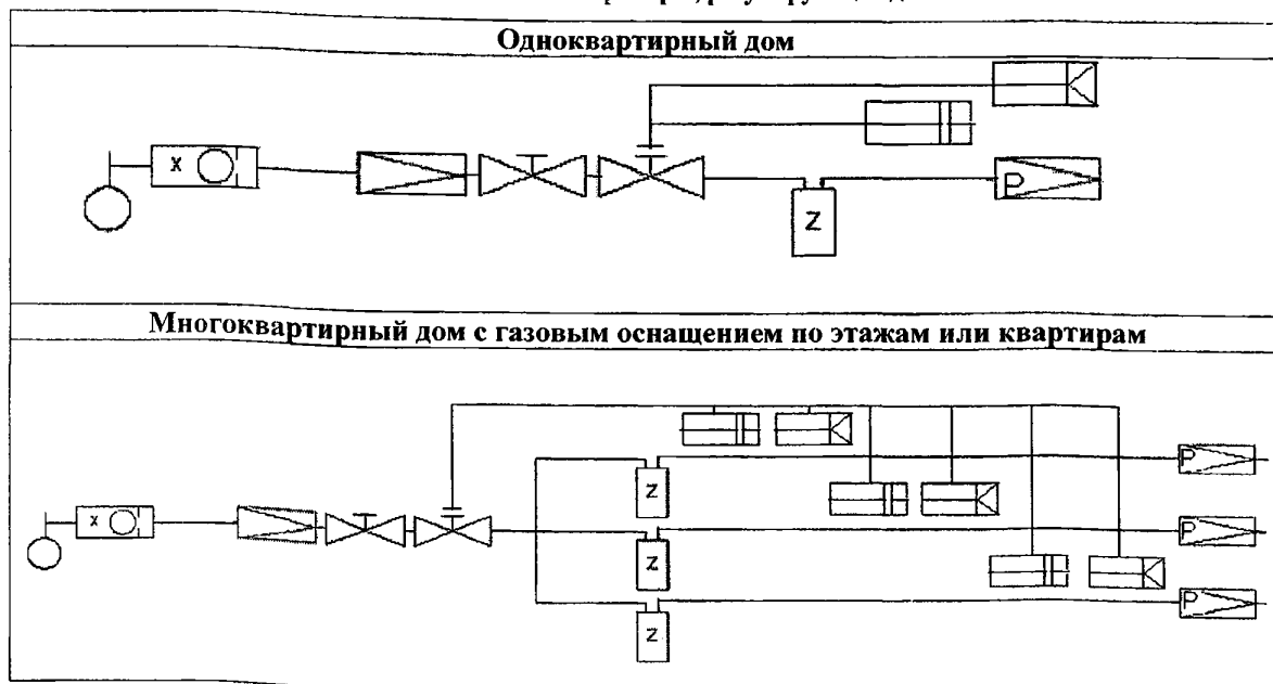
Рисунок Д.2 – Активные меры безопасности при давлении в наружном газопроводе свыше 0,005 МПа до 0,6 МПа включительно и приборы, регулирующие давление газа
