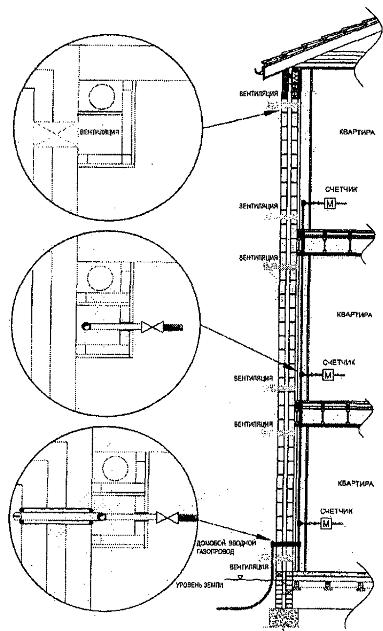
Рисунок Г.1 – Газопровод в вентилируемой штрабе
