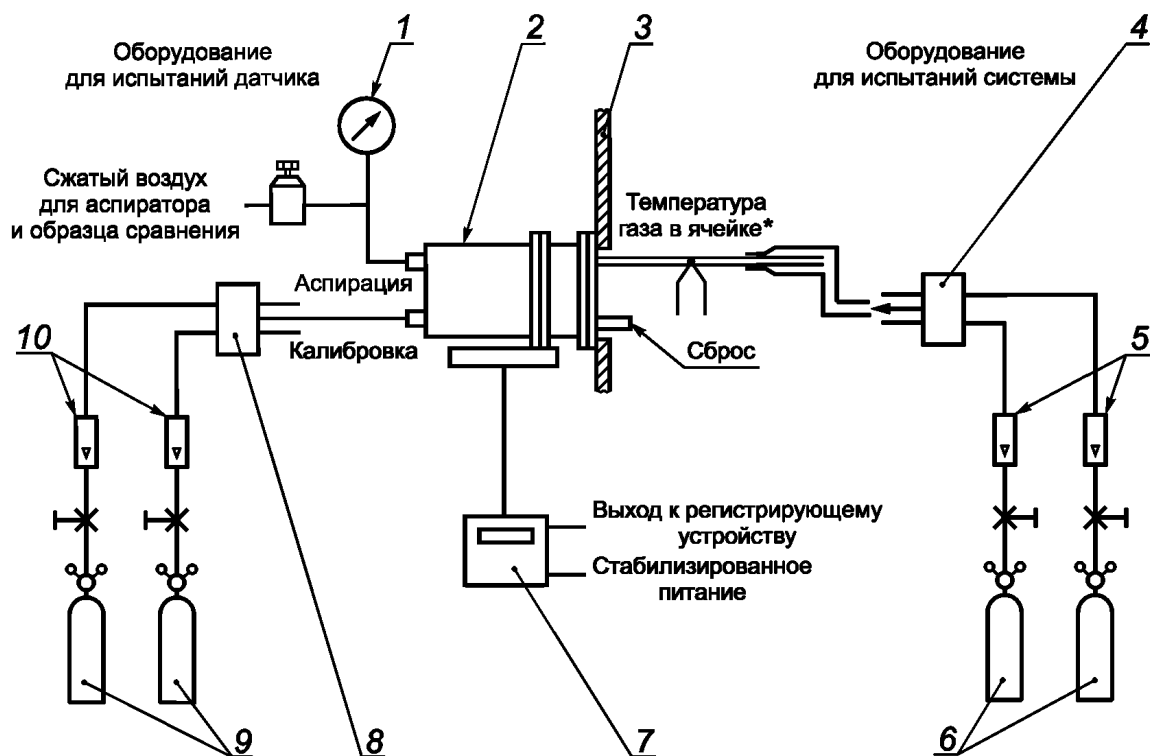
Рисунок 1 — Установка для определения динамических характеристик газоанализаторов «на месте»
