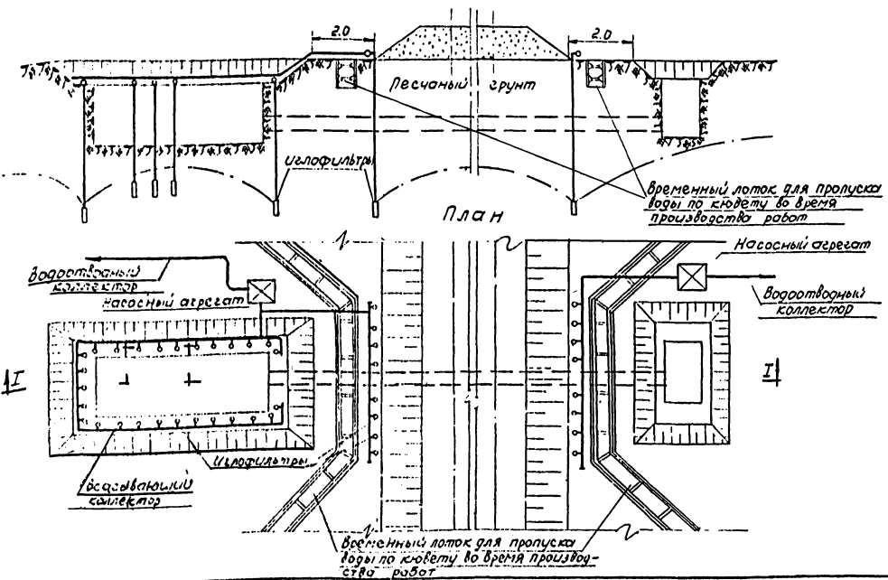
Разрез I-I
