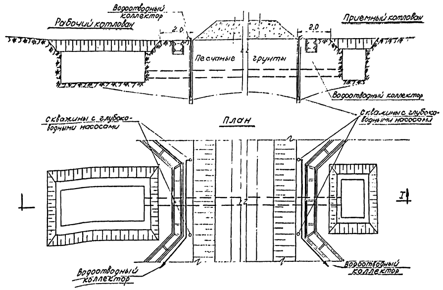
Разрез I-I
