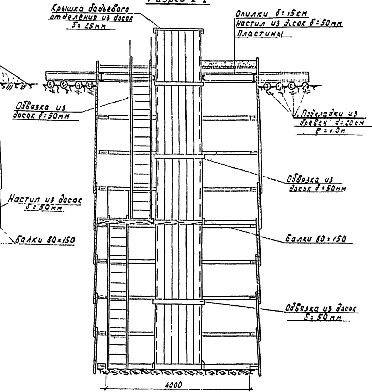
Разрез 2-2
