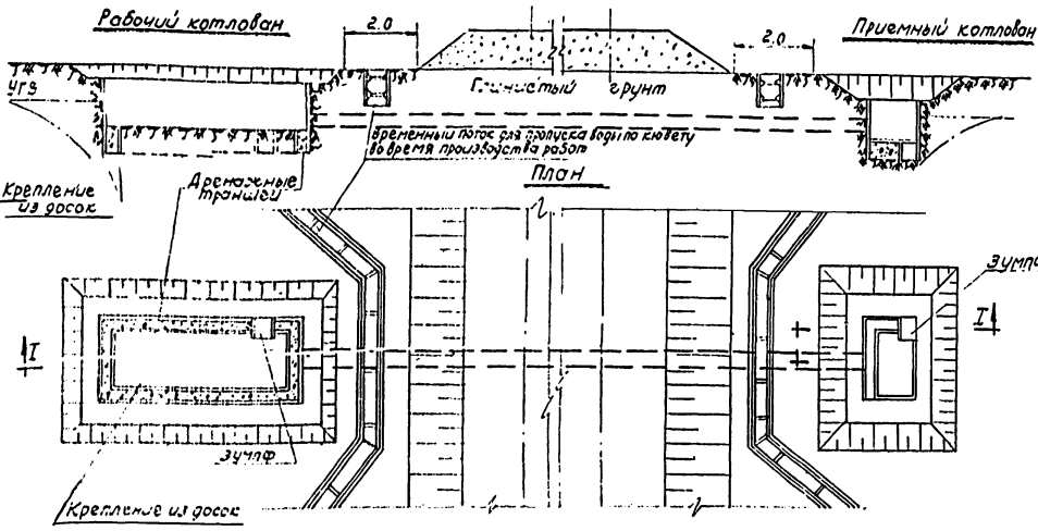
Разрез I-I
