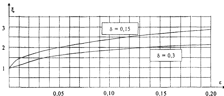
Рисунок 11.1 – Коэффициенты динамичности
