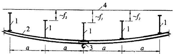
1 – стропильные конструкции; 2 – балка подвешного кранового пути; 3 – подвешной кран; 4 – исходное положение стропильных конструкций; f_1 – прогиб наиболее нагруженной стропильной конструкции; f_2 – прогибы смежных с наиболее нагруженной стропильных конструкций
