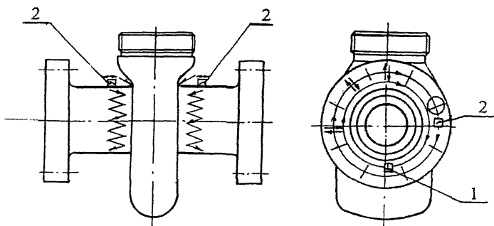
Рисунок Б.3 – Схема УЗД катушки
