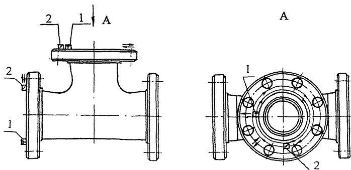
Рисунок Б.1 – Схема УЗД крестовика
