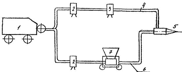
Рис. 1. Схема торкретной установки:
