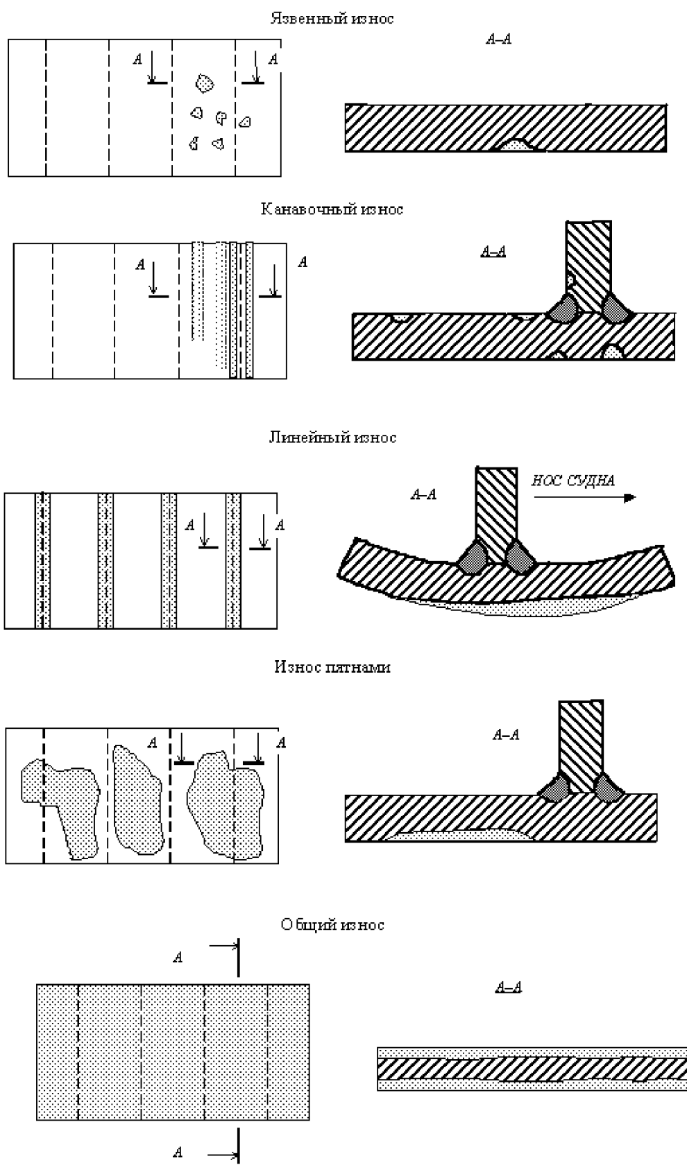
Рис. 1.2.1-2 Виды износов
