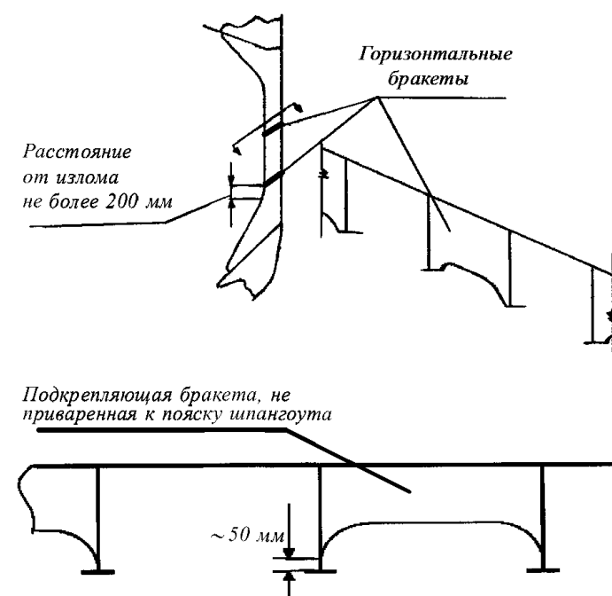
Рис. 5.12.3.3.1 Подкрепляющие brackets
