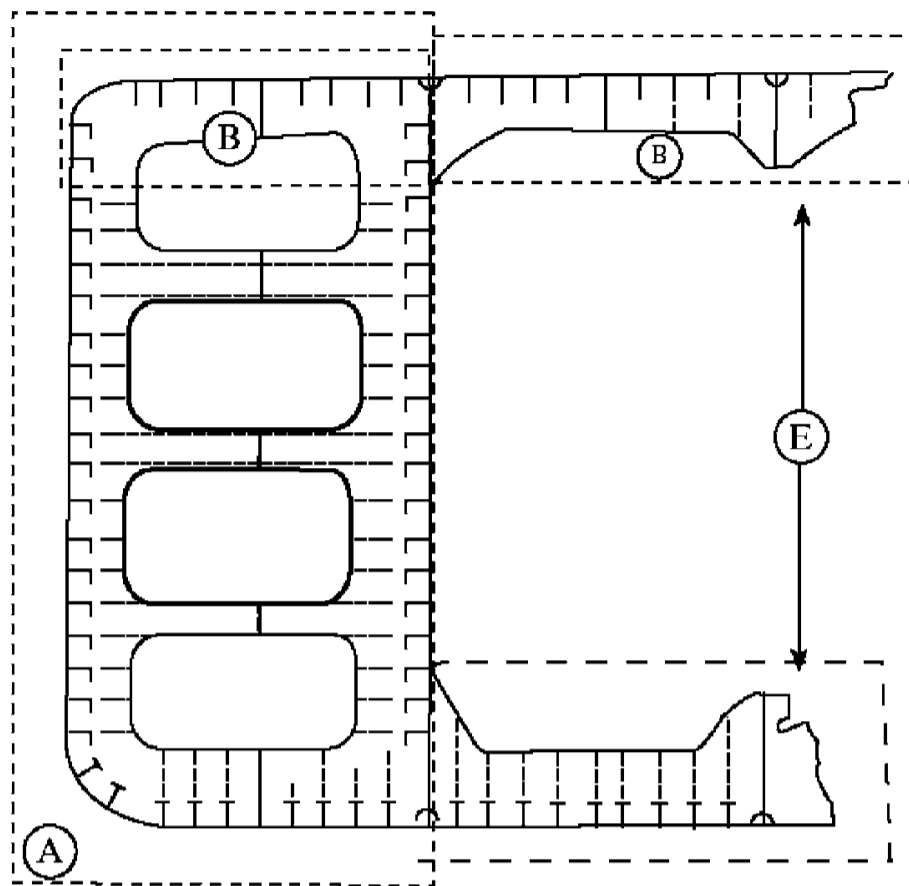
Типовое поперечное сечение химовоза Районы A, B и E детального освидетельствования
