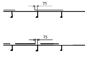
Рис. 5.2.2.4-1 Расположение накладных полос
