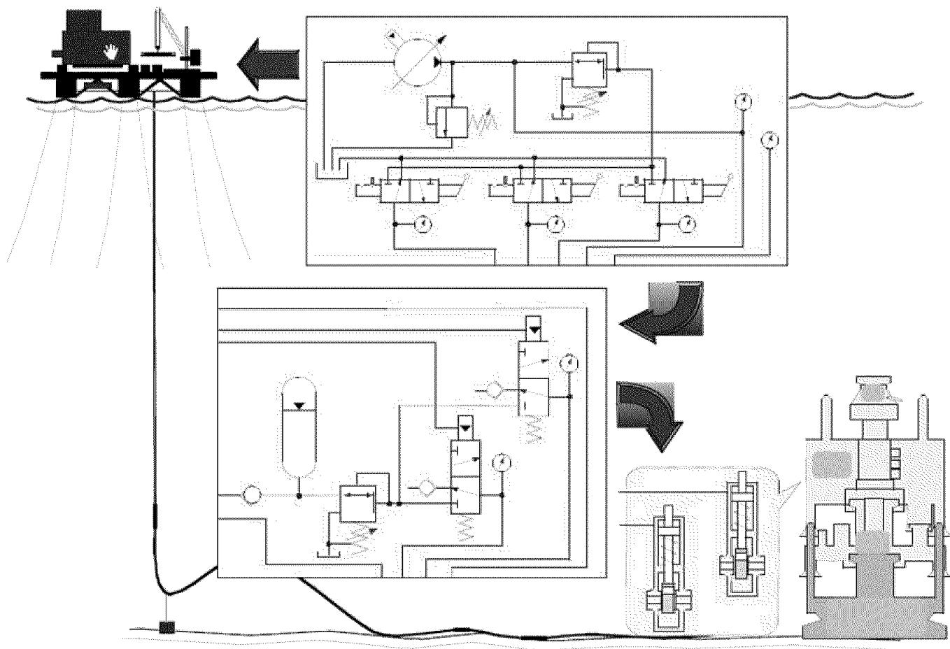
Рис. 3 Гидравлические системы с подводным управляющим модулем
