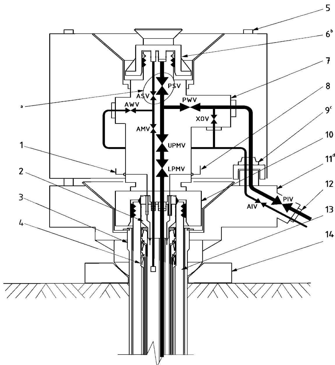
Рис. 1 Вертикальная устьевая арматура (VXT)
