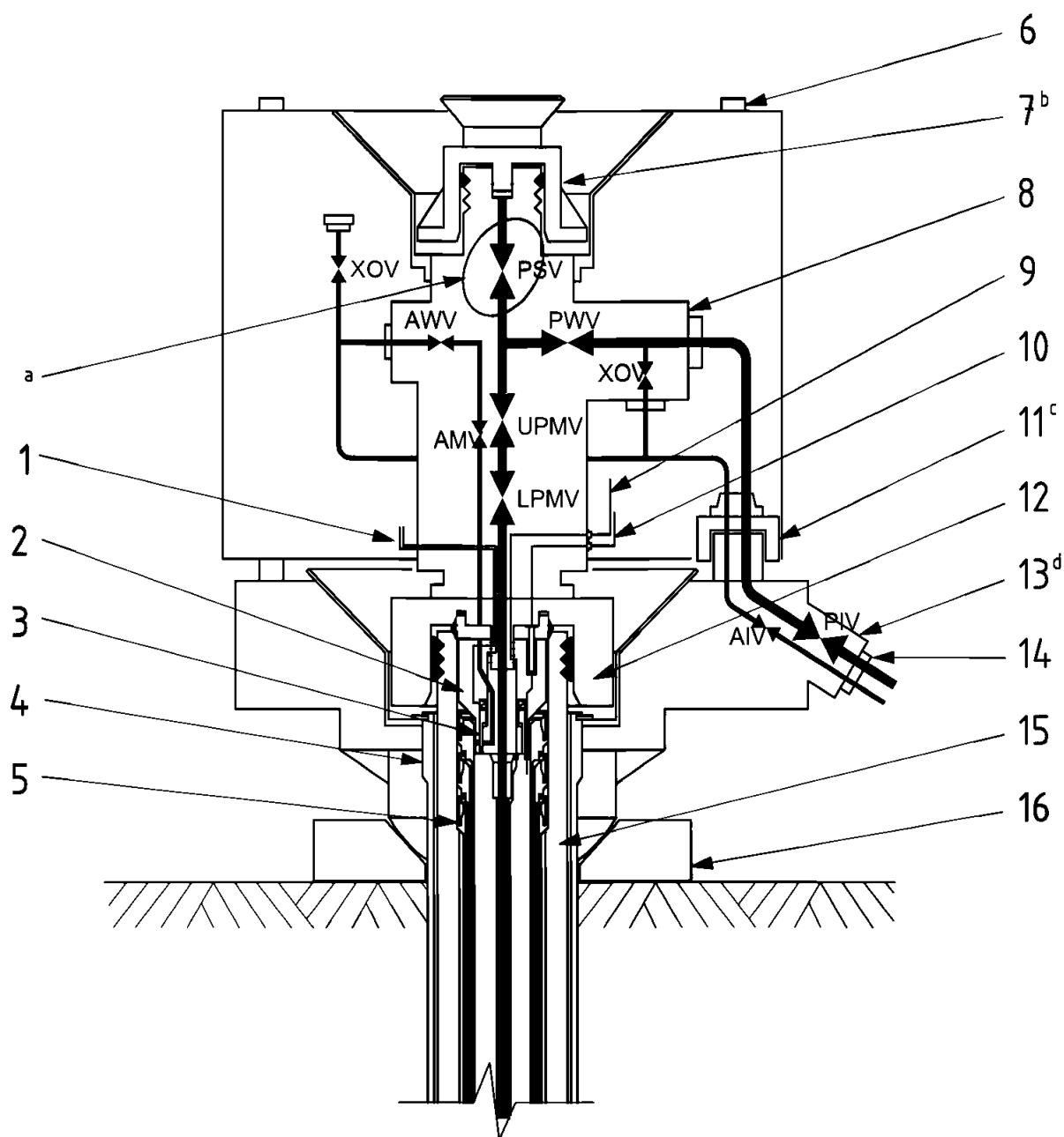
Рис. 3 Вертикальная устьевая арматура (VXT) концентрического типа
