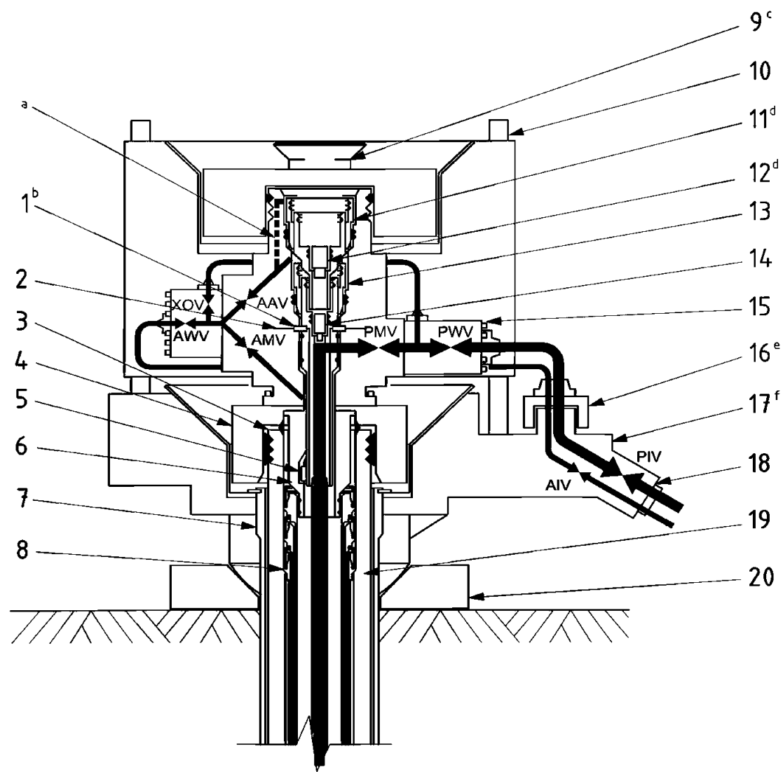
Рис. 5 Горизонтальная устьевая арматура (НХТ)
