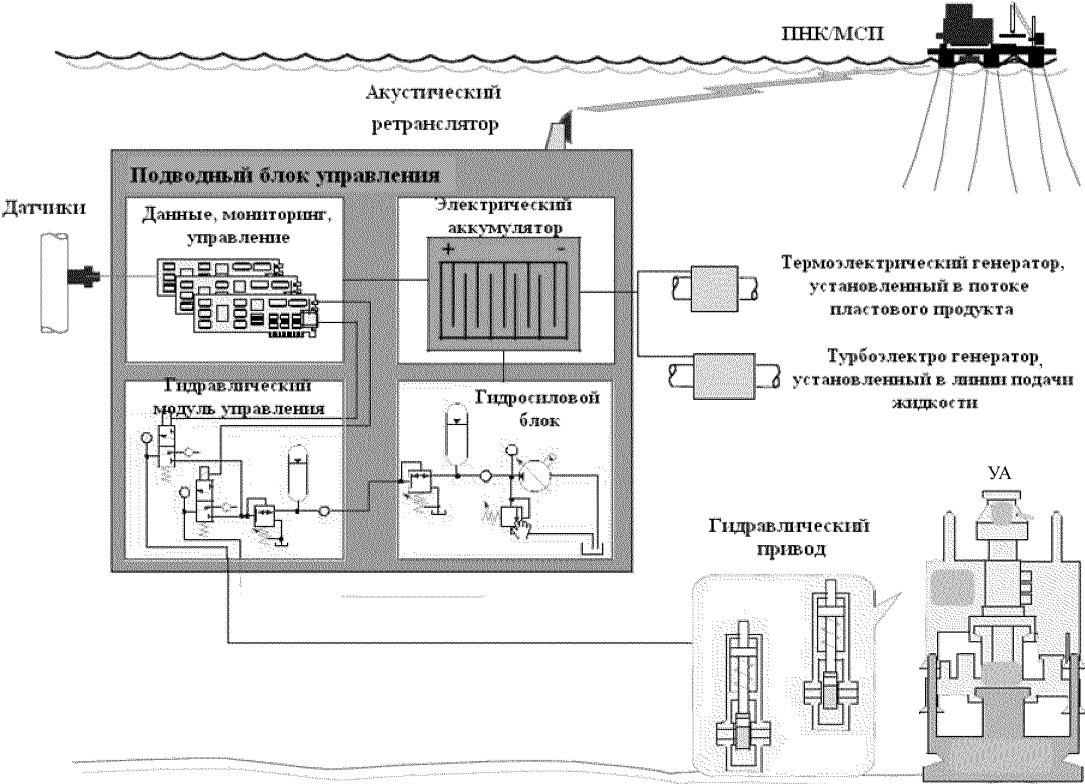
Рис. 7 Автономные системы (SPARCS)
