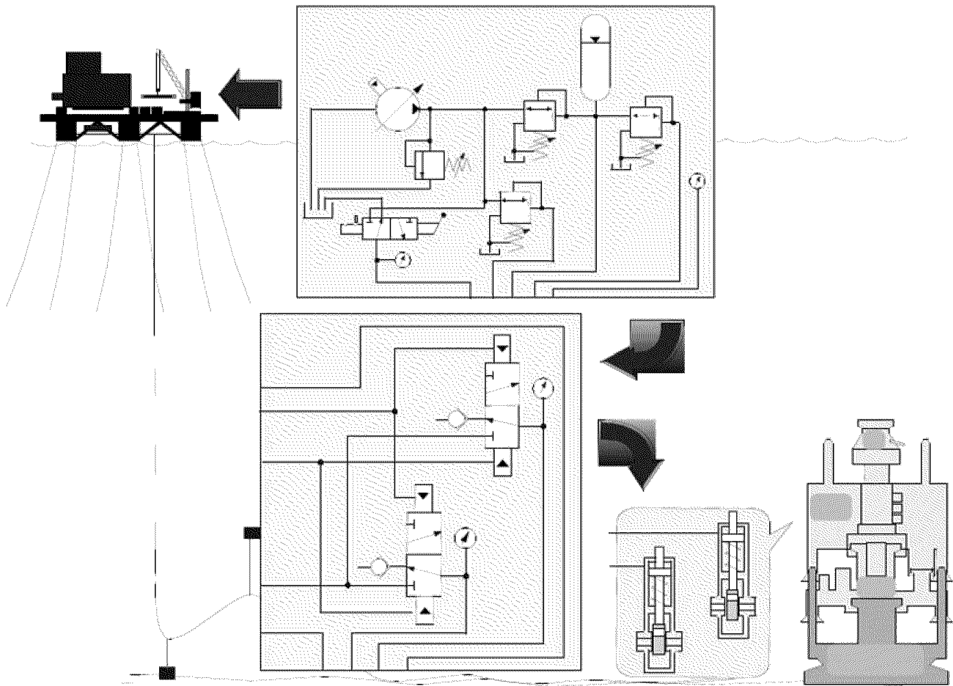
Рис. 4 Гидравлические системы с последовательным управлением
