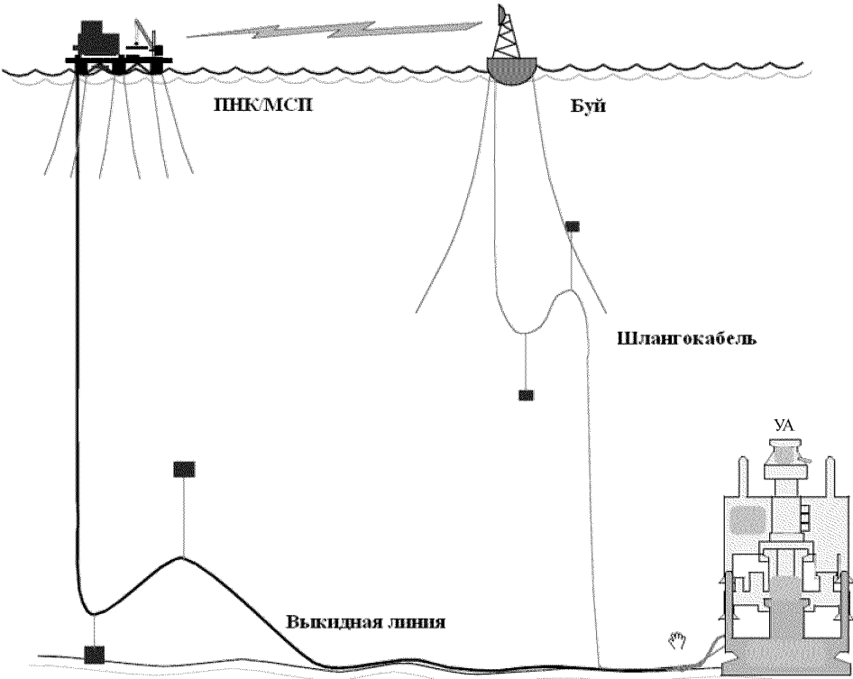
Рис. 8 Интегрированные буй контроля и управления (ICB)
