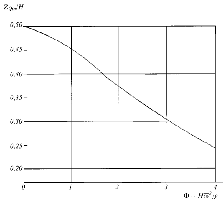
Рис. 3.1.4.13-3 Зависимость Z_{Qin}/H от параметра \Phi = H\omega^2/g
