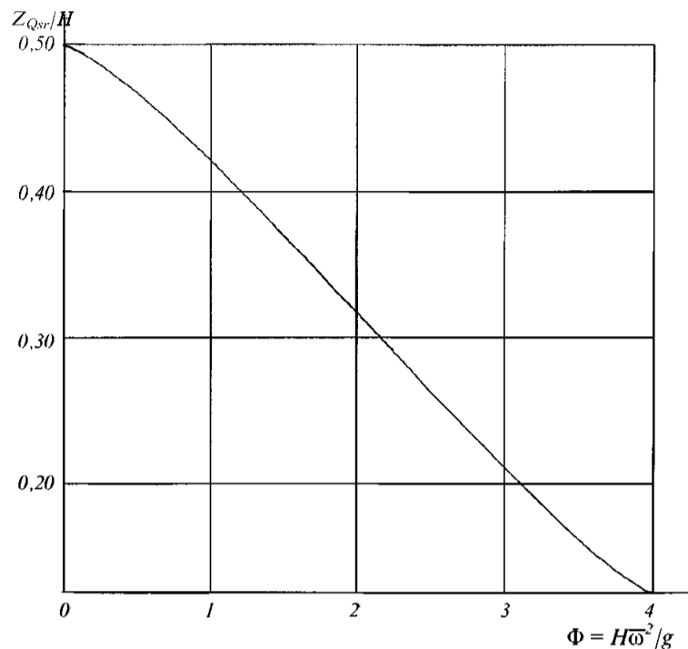
Рис. 3.1.4.13-2 Зависимость Z_{Qsr}/H от параметра \Phi = H\omega^2/g
