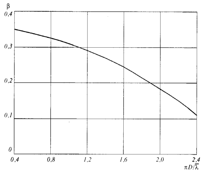
Рис. 3.3.2.1.8.2 Зависимость коэффициента \beta от \pi D / \lambda
