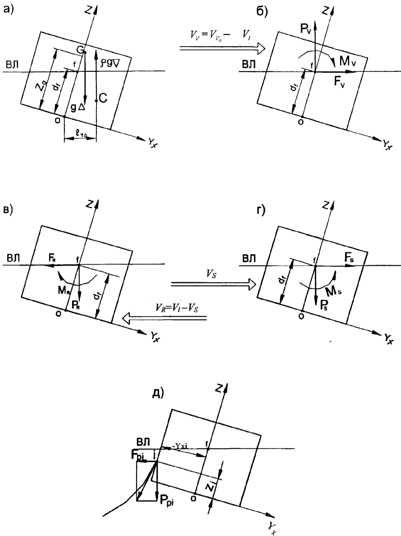
Рис. 2.3.2 Схемы внешних воздействий в плоскости наклонения объекта
