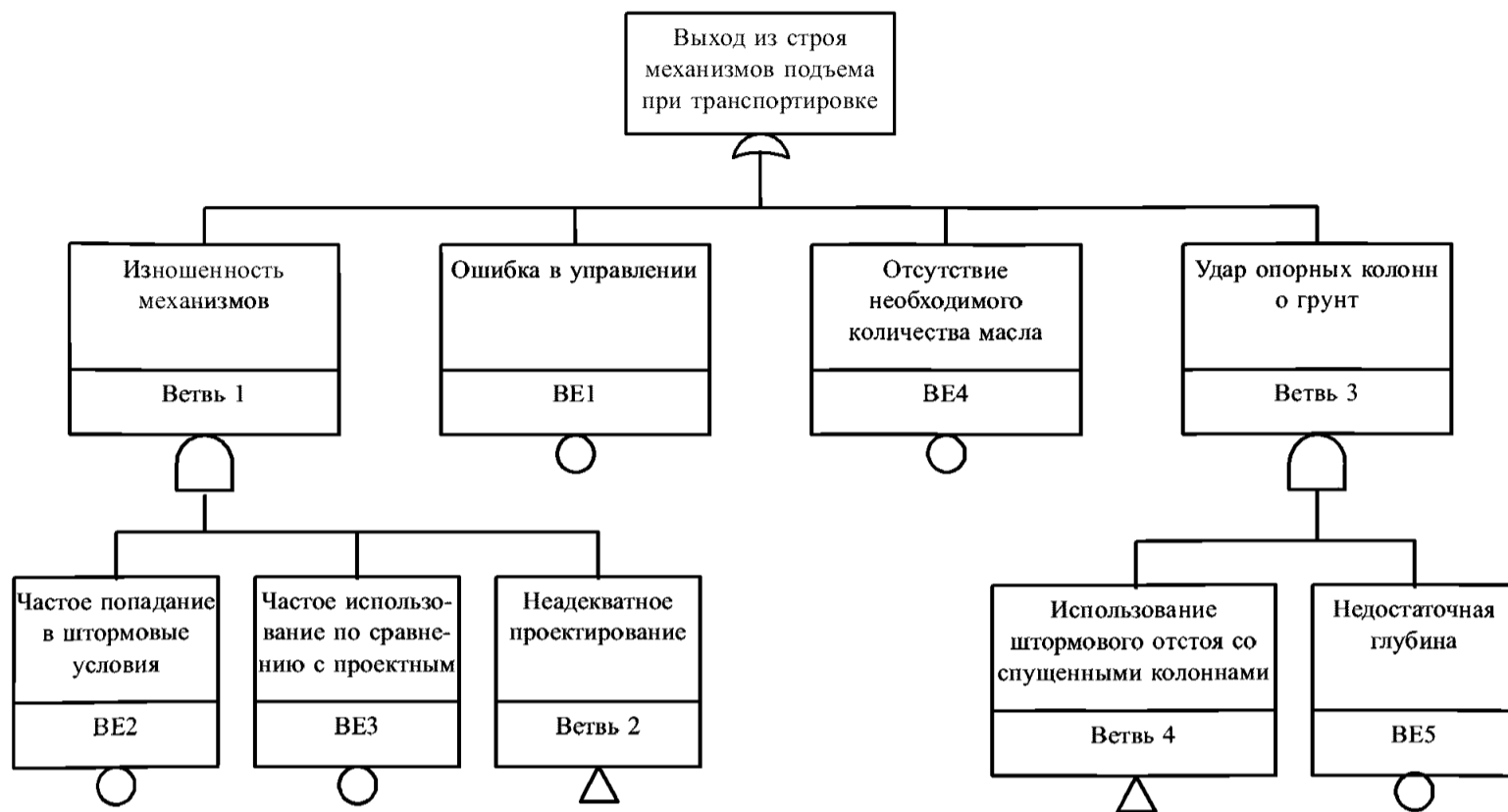
Начальное построение дерева ошибок и неполадок
