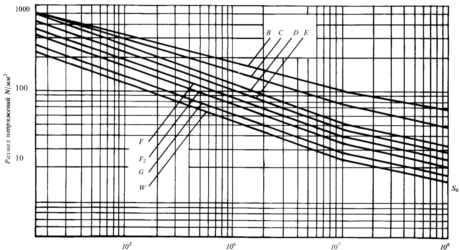
Рис. 2.4.4.8-1 Кривые усталости
