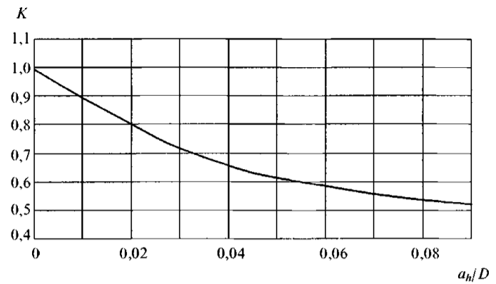
Рис. 3.3.2.3.3-1 Параметр формы K в зависимости от a_h/D
