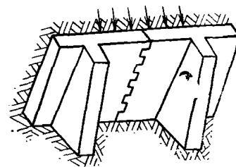
Рис. 3. Растяжение кладки при изгибе по перевязанному сечению
