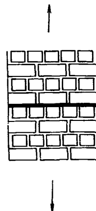
Рис. 1. Растяжение кладки по неперевязанному сечению
