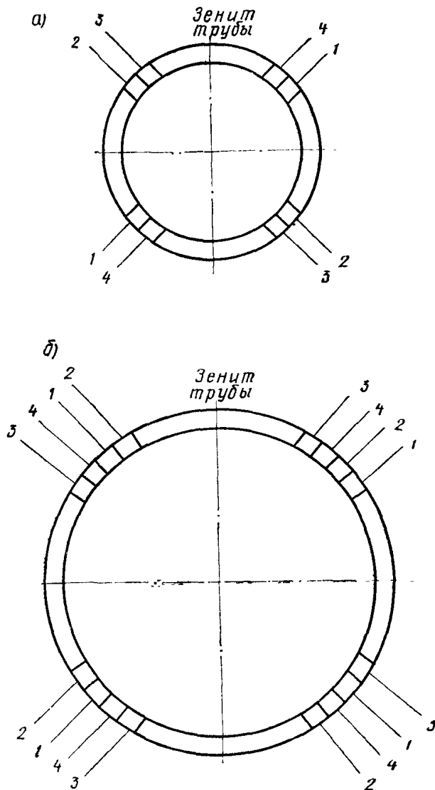
Рис. 1. Схема вырезки образцов для механических испытаний
