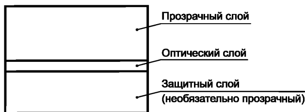
Рисунок 1 — Поперечное сечение карты в оптической зоне
