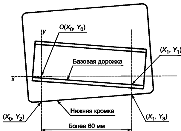
Рисунок 3 — Метод измерения наклона
