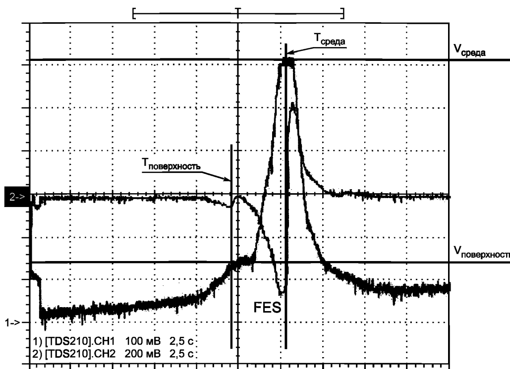
Рисунок 6 — Формы сигналов, получаемые при развертке по фокусу
