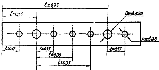
1й вариант простановки размеров
