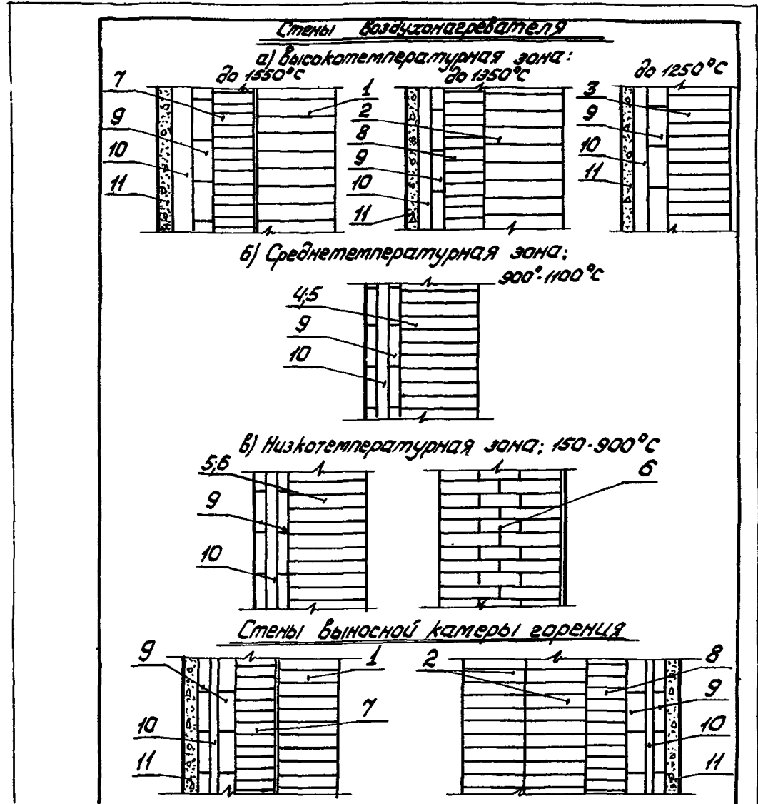
Рис.39. Кладка стен воздухоподогревателя и выносной камеры горения: 1 - диасовые изделия ДВ; 2 - высокоглиноземистые муллитокорундовые изделия (МКВ-72); 3 - высокоглиноземистые муллитовые изделия (МЛВ-62); 4 - шамотные изделия ШВ-42; 5 - шамотные изделия ШВ-37; 6 - шамотные изделия ШВ-28; 7 - диас легковесный; 8 - каолиновый легковес; 9 - шамот легковесный; 10 - муллитокремнеземистые волокнистые изделия; 11 - торкрет-масса
