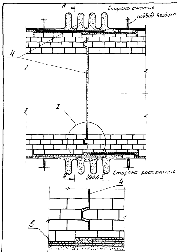
Рис. 54 Кладка воздухопровода горячего дутья в районе компенсатора 1- высокоглиноземистые муллитокорундовые изделия (МКЖ-72) 2- каменные легкие изделия КЛ-1,3 3- шамотные легкие изделия ШЛ-1,4 4- высокоглиноземистая бета 5- асбестовый картон
