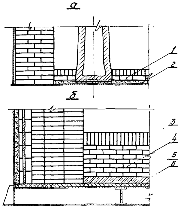
Рис.38. Кладка дна: а - камеры насадки; б - выносной камере горения; 1 - шамотные изделия ШВ-28; 2 - шамотно-глинисто-цементный раствор; 3 - высокоглиноземистые муллитокорундовые изделия (МКВ-72); 4 - шамотные легковесные изделия; 5 - муллитокремнеземистые волокнистые изделия; 6 - асбестовый картон
