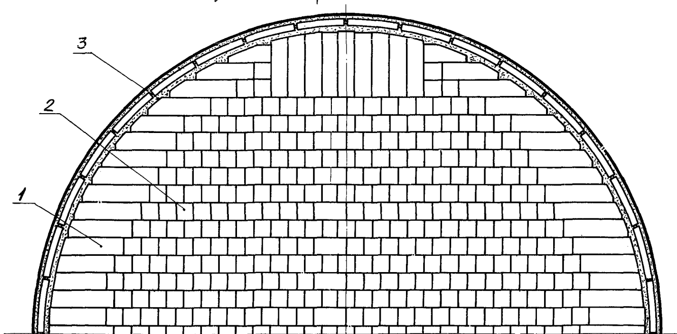
Рис.4. Комбинированная кладка лещади и горна. План графитированных блоков: 1 - горизонтальные графитированные блоки; 2 - вертикальные графитированные блоки; 3 - углеродистая масса
