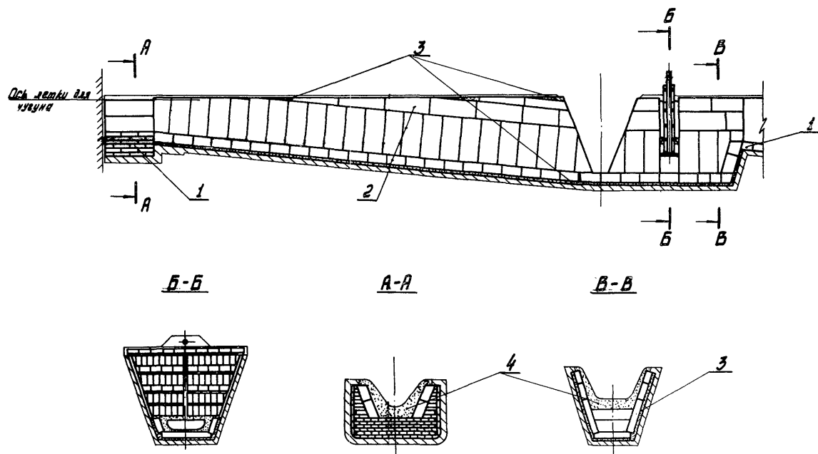
Рис. 59. Кладка главного желоба углеродистыми блоками и шамотными изделиями
