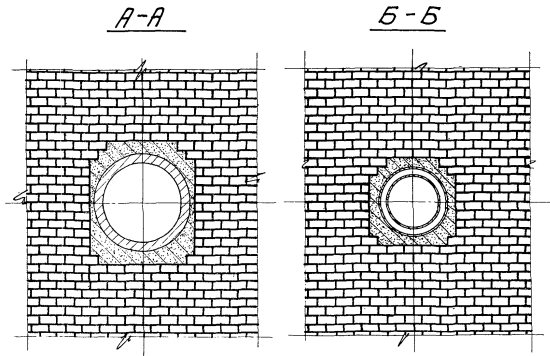
Рис.15. Кладка в районе воздушных фурт:
