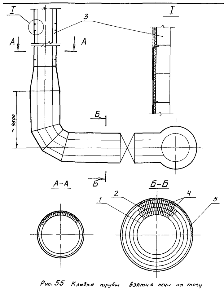
Рис.55. Кладка трубы взятия печи на тягу: 1 - муллитокорундовые изделия МКВ-72; 2 - муллитовые изделия МЛВ-62; 3 - шамотные изделия; 4 - шамотные легковесные изделия; 5 - асбестовый картон
