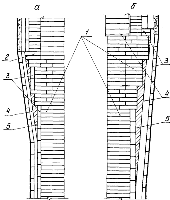
Рис. 40. Кладка стен воздухонагревателя в районе расширения кожуха:
