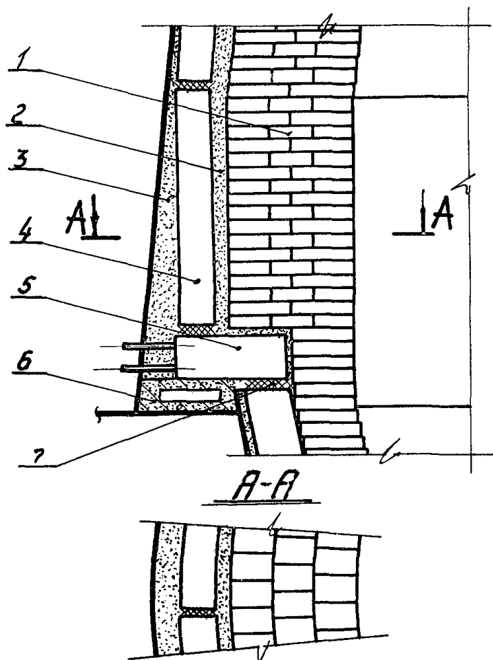
Рис.18. Кладка толстостенного распара с периферийными плитовыми холодильниками: 1 - шамотные каолиновые изделия; 2 - углеродистая масса; 3 - шамотно-глинисто-цементный раствор; 4 - периферийные плитовые холодильники; 5 - мараторные холодильники; 6 - шамотно-глинистая масса; 7 - чугунная замазка
