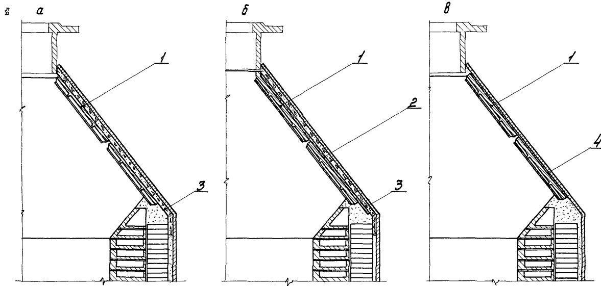
Рис.34. Футеровка купола печи.
