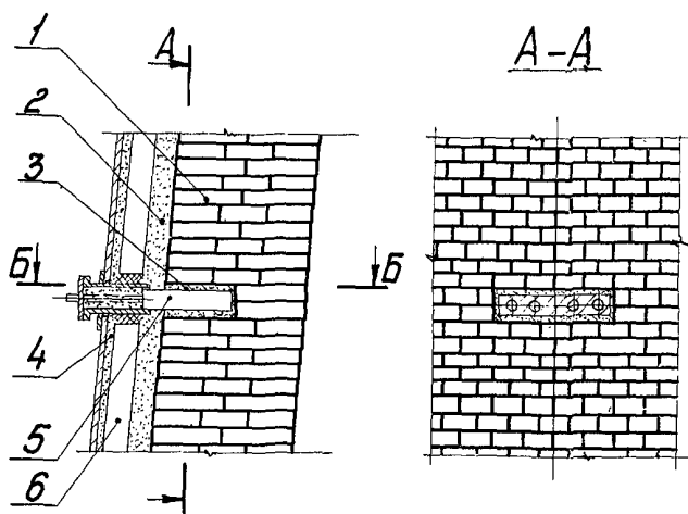
Рис.20. Кладка шахты вокруг сменяемых горизонтальных холодильников с амбразурами в сочетании с периферийными плитовыми холодильниками: 1 - шамотные каолиновые изделия; 2 - углеродистая масса; 3 - шамотно-глинистая масса; 4 - шамотно-глинисто-цементный раствор; 5 - горизонтальный холодильник; 6 - периферийные плитовые холодильники
