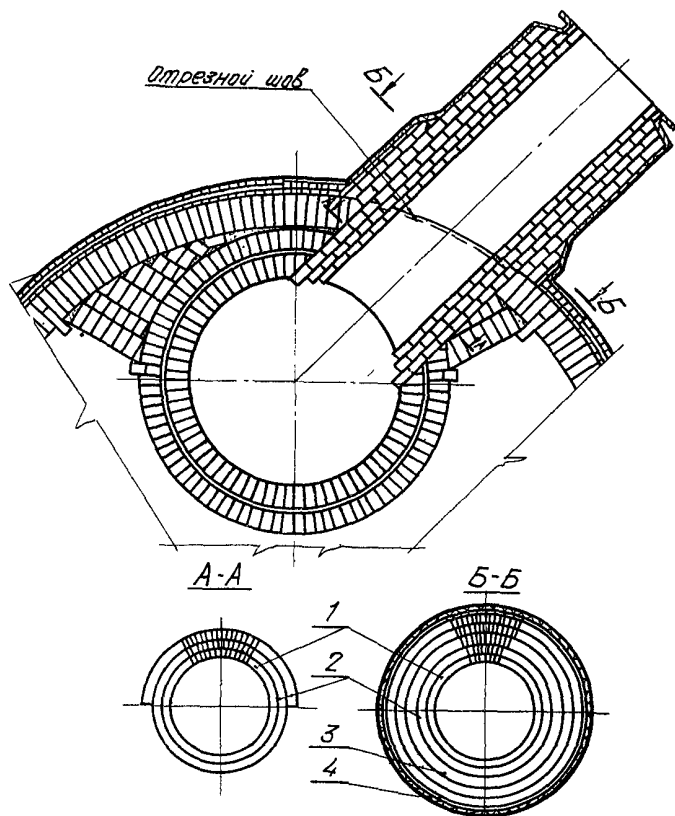
Рис.49. Кладка штулера клапана горячего дутия: 1 - муллитокорундовые изделия МКВ-72; 2 - шамотные изделия или муллитовые МЛВ-62; 3 - шамотные легковесные изделия; 4 - асбе- стовый картон
