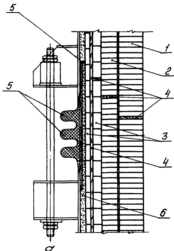
Рис.42. Кладка камеры горения в районе компенсатора:
