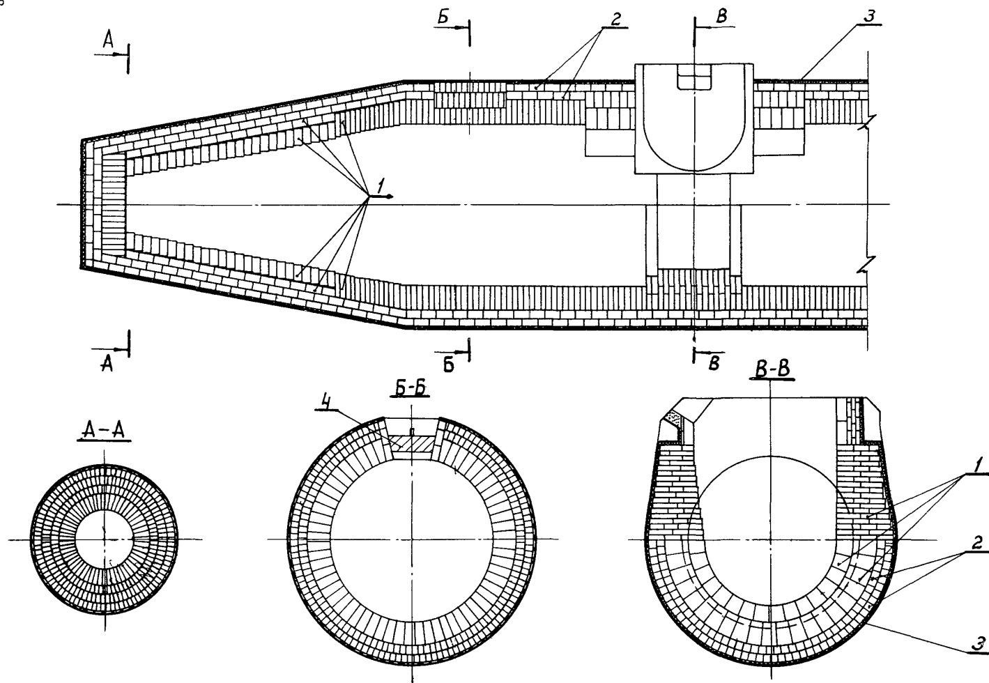
Рис. 63. Кладка чугуновозного котла миксерного типа емкостью 420 т
