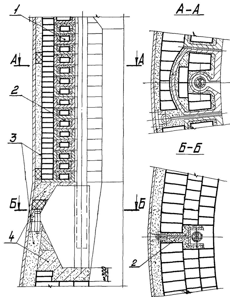
Рис.32. Кладка в районе установки приемника излучения УРМС: 1 - шамотные изделия; 2 - шамотно-глинистая масса; 3 - шлако-асбестовая масса; 4 - глинисто-асбестовая масса
