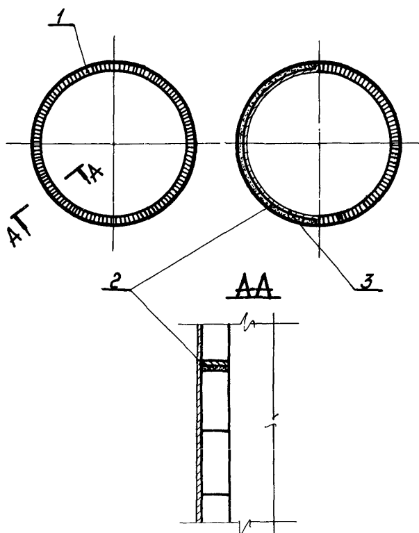
Рис. 57. Кладка газопровода грязного газа.
