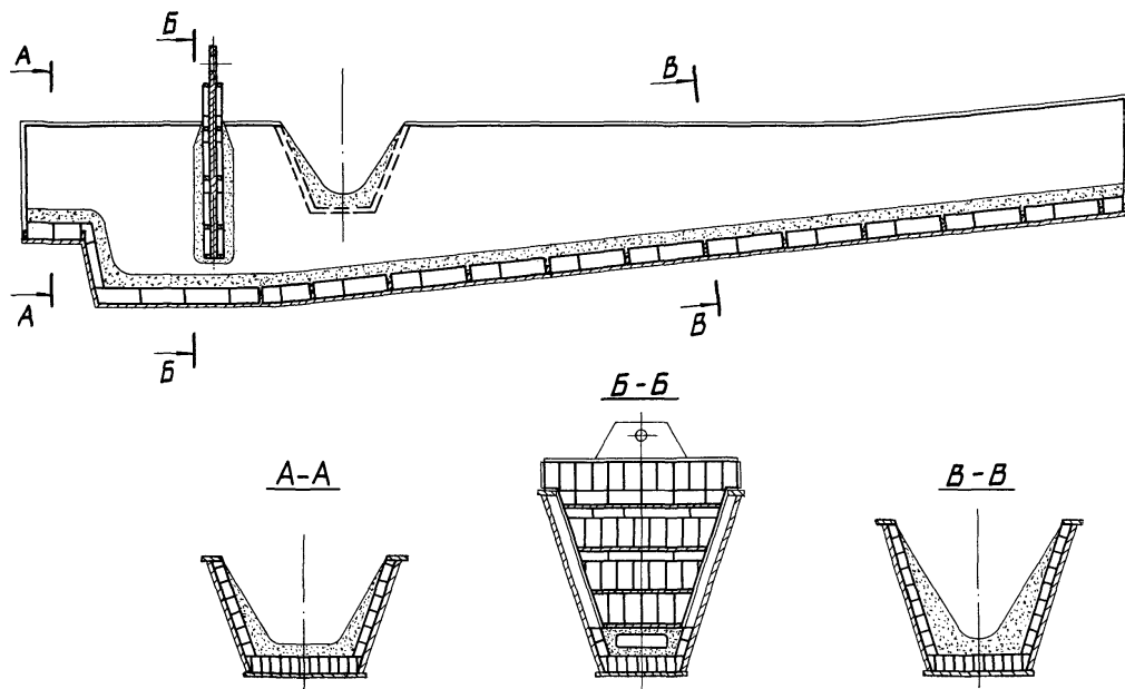
рис. 60. Кладка главного сменного желоба: 1- шамотные изделия; 2- набивная огнеупорная масса.
