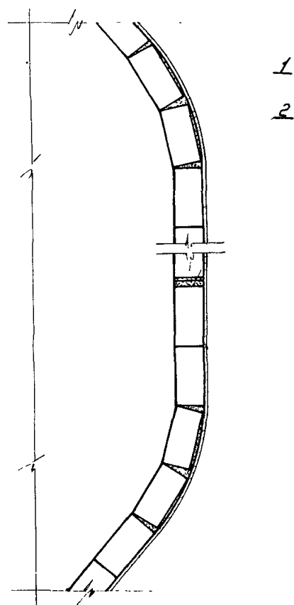
Рис.56. Кладка пылеуловителя: 1 - шамотные изделия ШБ-1; 2 - шамотно-глинисто-цементный раствор
