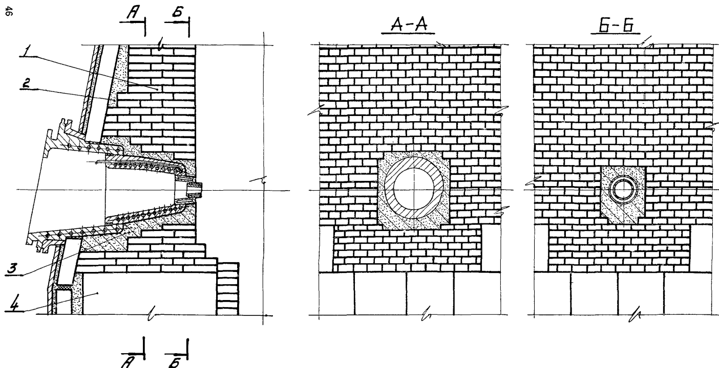
Рис. 14. кладка в районе летки для шлака:
