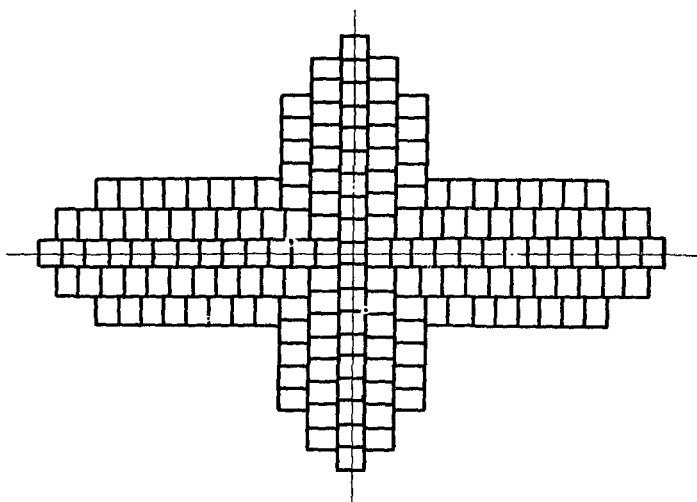
Рис.6. Закладка деревянного креста при кладке алмосиликатной части лещадки: 1 - ось печи; 2 - шнур; 3 - брус
