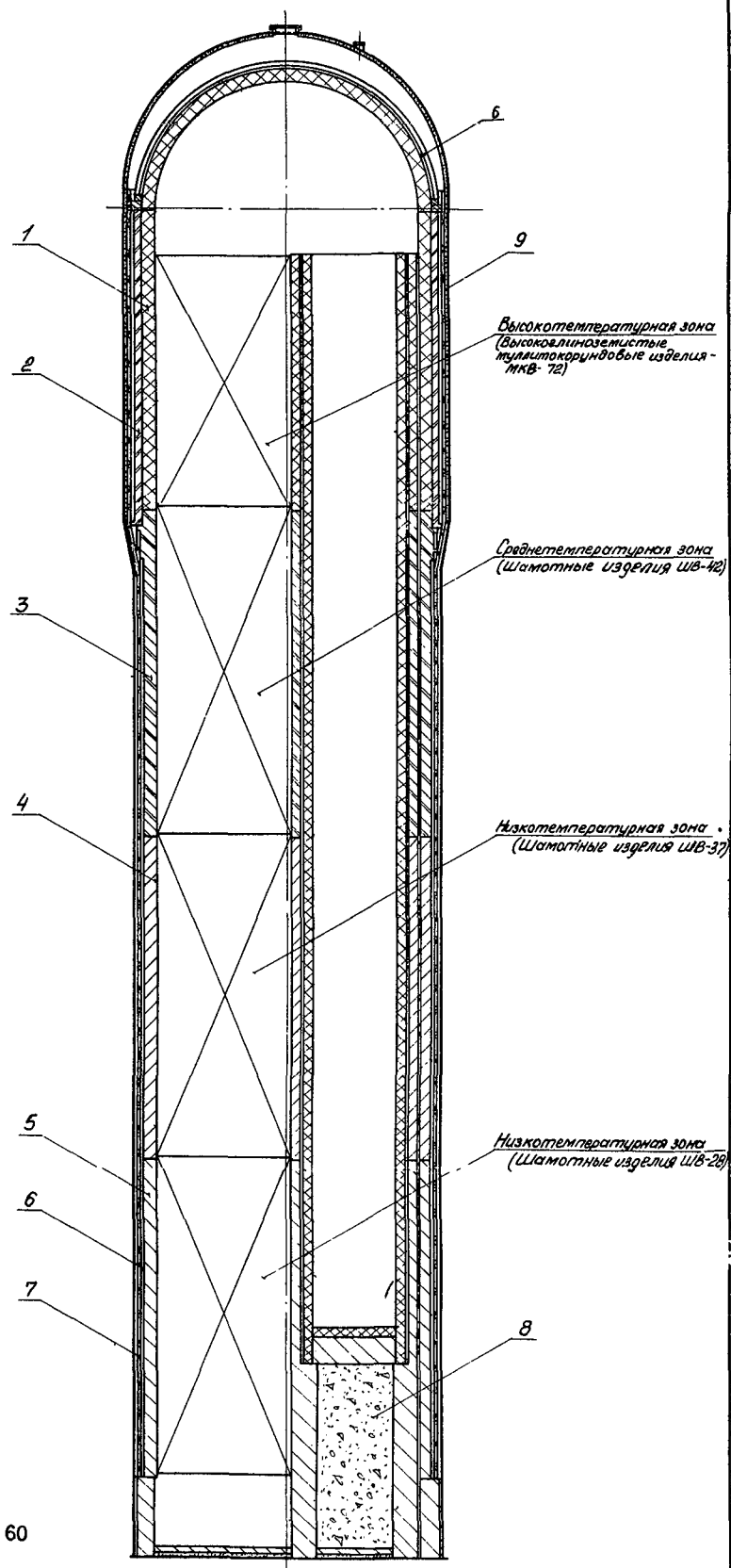
Рис.36. Распределение огнеупоров в кладке воздушонагревателя с температурой под куполом до 1350^{\circ}\text{C} : 1 - высокоглиноземистые мулито-корундовые изделия (МКВ-72); 2 - каолиновый легковес; 3 - шамотные изделия ШВ-42; 4 - шамотные изделия ШВ-37; 5 - шамотные изделия ШВ-28; 6 - шамот легковесный; 7 - мулито-кремнеземистые волокнистые изделия; 8 - бой обыкновенного глиняного кирпича; 9 - торкрет-масса
