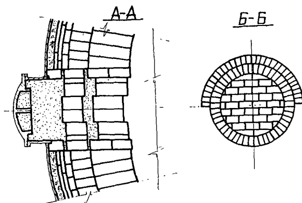
Рис.52. Кладка лаза в подкупольном пространстве 1 - высокоглиноземистые муллитокорундовые изделия;
