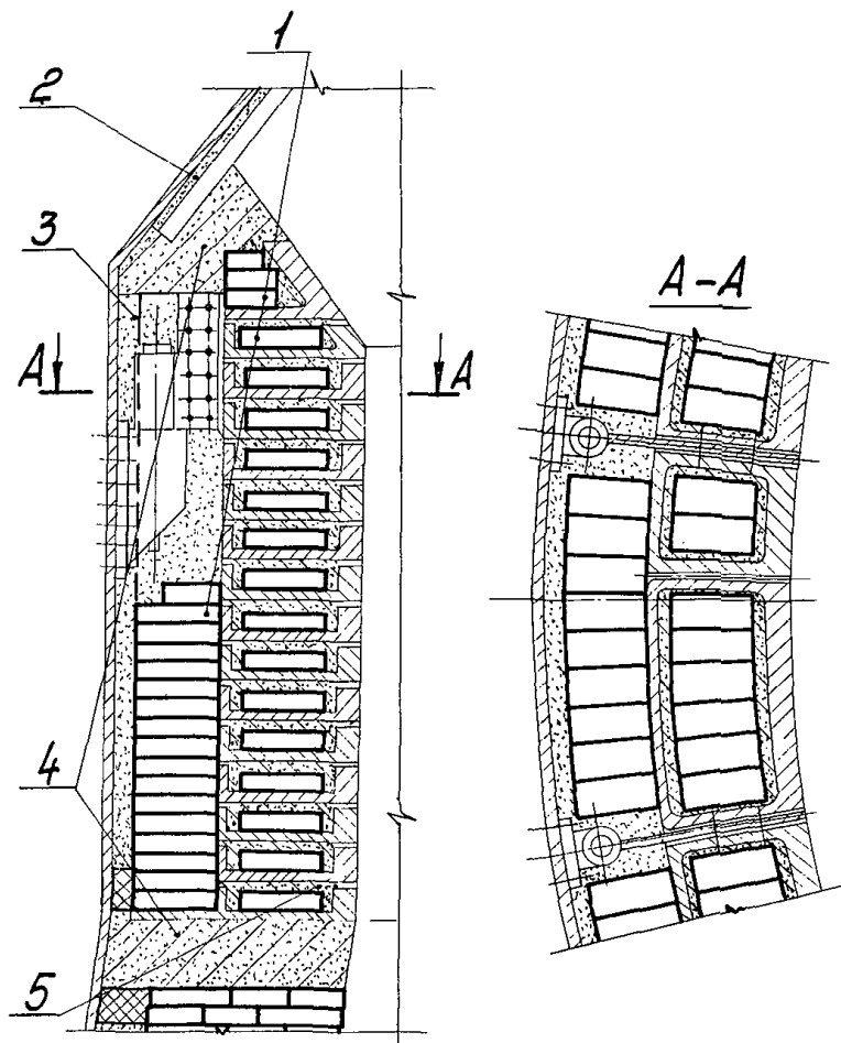
Рис.30. Кладка в районе футеровочных плит колошника. Вариант II: 1 - шамотные изделия; 2 - шамотно-цементный раствор; 3 - шлако-асбестовая масса; 4 - глинисто-асбестовая масса; 5 - шамотно-глинистая масса
