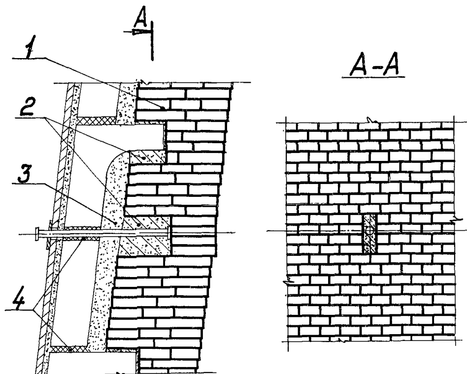
Рис.24. Кладка глухих отверстий для термопар шахты: 1 - шамотные каолиновые изделия; 2 - шамотно-глинистая масса; 3 - углеродистая масса; 4 - чугунная замазка
