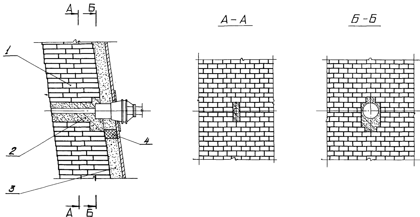
Рис. 26. Кладка отверстий в шахте для установки машины для отбора проб газа:
