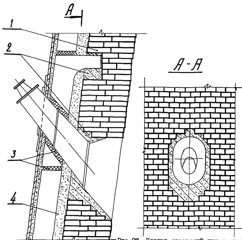
Рис.27. Кладка отверстий для установки устройств для измерения статического давления газа в шахте: 1 - шамотные каолиновые изделия; 2 - шамотно-глинистая масса; 3 - чугунная закладка; 4 - углеродистая масса
