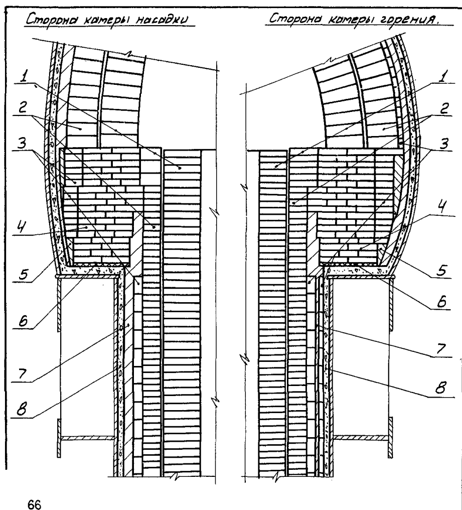
Рис.45. Кладка купола воздухонагревателя с выносной камерой горения: 1 - диасовые изделия ЛВ; 2 - диас легковесный; 3 - шамот легковесный; 4 - высокоглиноземистые муллитокорундовые изделия (МКВ-72); 5 - вата высокоглиноземистая; 6 - асбестовый картон; 7 - муллитокремнеземистые волокнистые изделия; 8 - торкрет-масса
