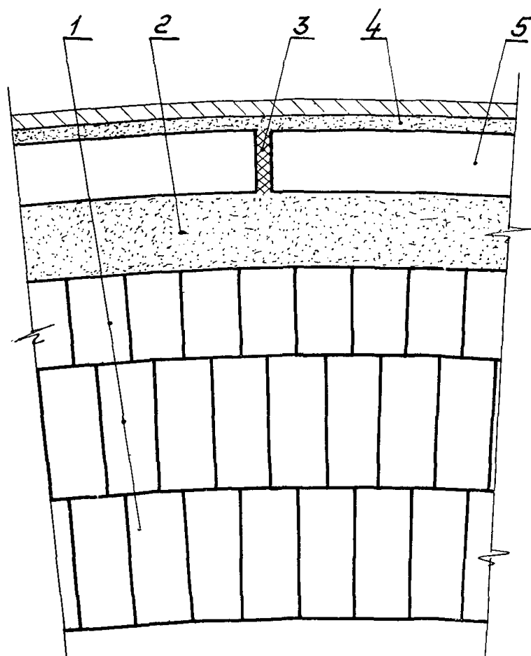
Рис.11. Кладка стен горна шамотными каолиновыми изделиями. План. 1 - шамотные каолиновые изделия; 2 - углеродистая масса; 3 - чугунная замазка; 4 - шамотно-глинисто-цементный раствор; 5 - периферийные плитовые холодильники
