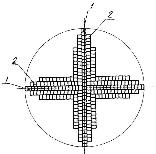
Рис.7. Кладка алмосиликатной части ле- щадки с нормальным количеством штраб: 1 - луч креста; 2 - нитка
