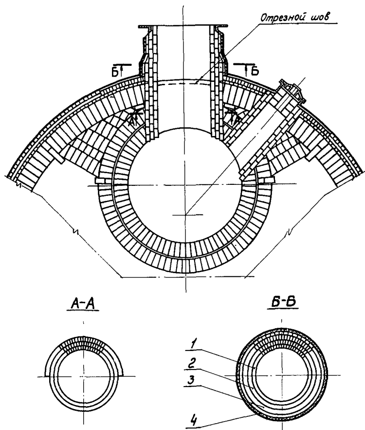
Рис.50. Кладка штуцера газовой горелки и лаза с люком для зажигания : 1 - высокоглиноземистые муллитокорундовые (МКВ-72) или муллитовые (МЛВ-62); 2 - шамотные изделия; 3 - шамотные легкие изделия; 4 - асбестовый картон
