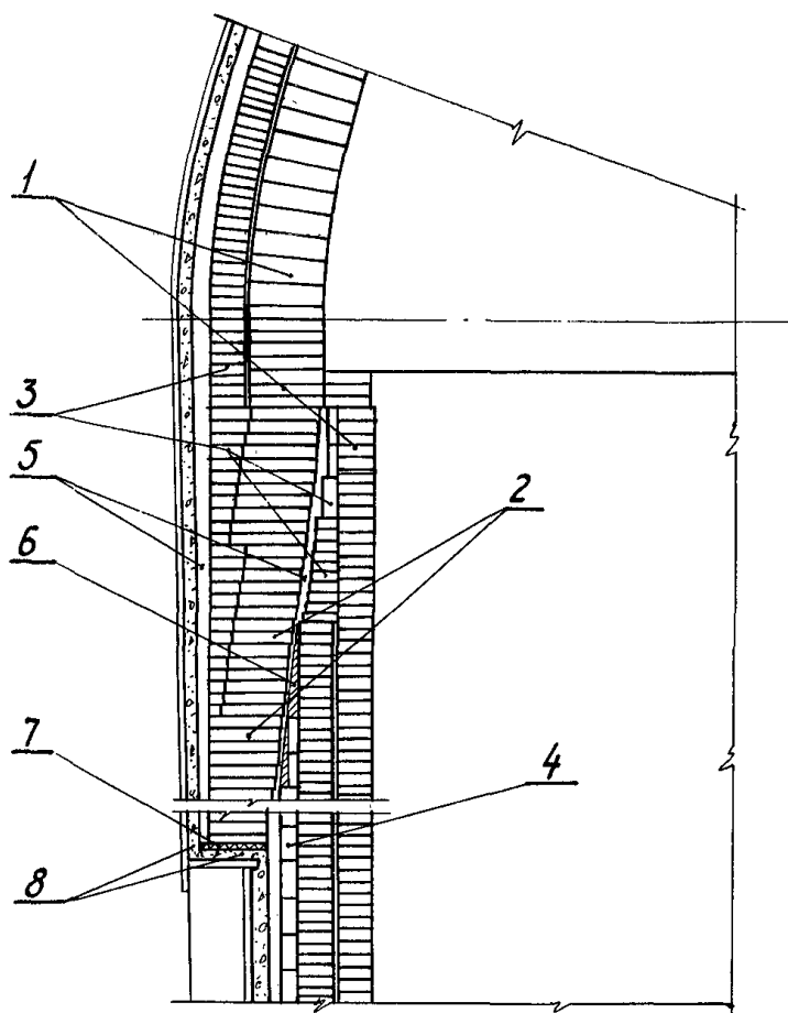
Рис.44. Кладка купола воздухонагревателя с опиранием на самостоятельную опору: 1 - диасовые изделия; 2 - шамотные каолиновые изделия; 3 - диасовые легковесные изделия; 4 - шамотные легковесные изделия; 5 - муллитокремнеземистые волокнистые изделия; 6 - высокоглиноземистая вата; 7 - асбестовый картон; 8 - торкрет-масса
