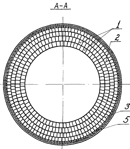
Рис. 54 Кладка воздухопровода горячего дутья в районе компенсатора 1- высокоглиноземистые муллитокорундовые изделия (МКЖ-72) 2- каменные легкие изделия КЛ-1,3 3- шамотные легкие изделия ШЛ-1,4 4- высокоглиноземистая бета 5- асбестовый картон
