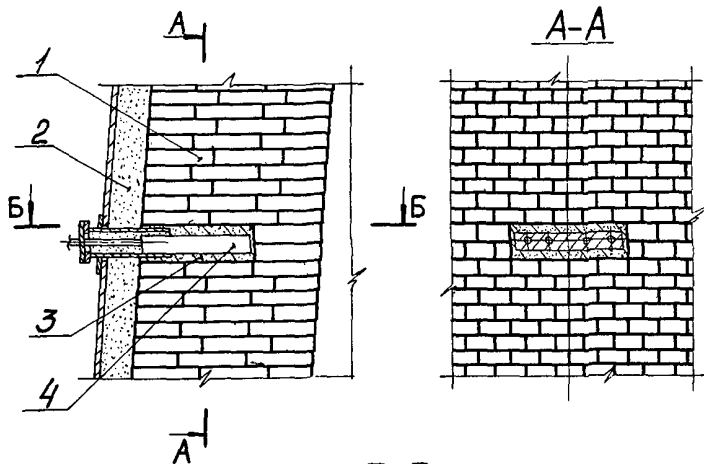
Рис.21. Кладка шахты вокруг сменяемых горизонтальных холодильников с амбразурами: 1 - шамотные каолиновые изделия; 2 - шамотно-асбестовая или шлакоасбестовая масса; 3 - шамотно-глинистая масса; 4 - горизонтальный холодильник
