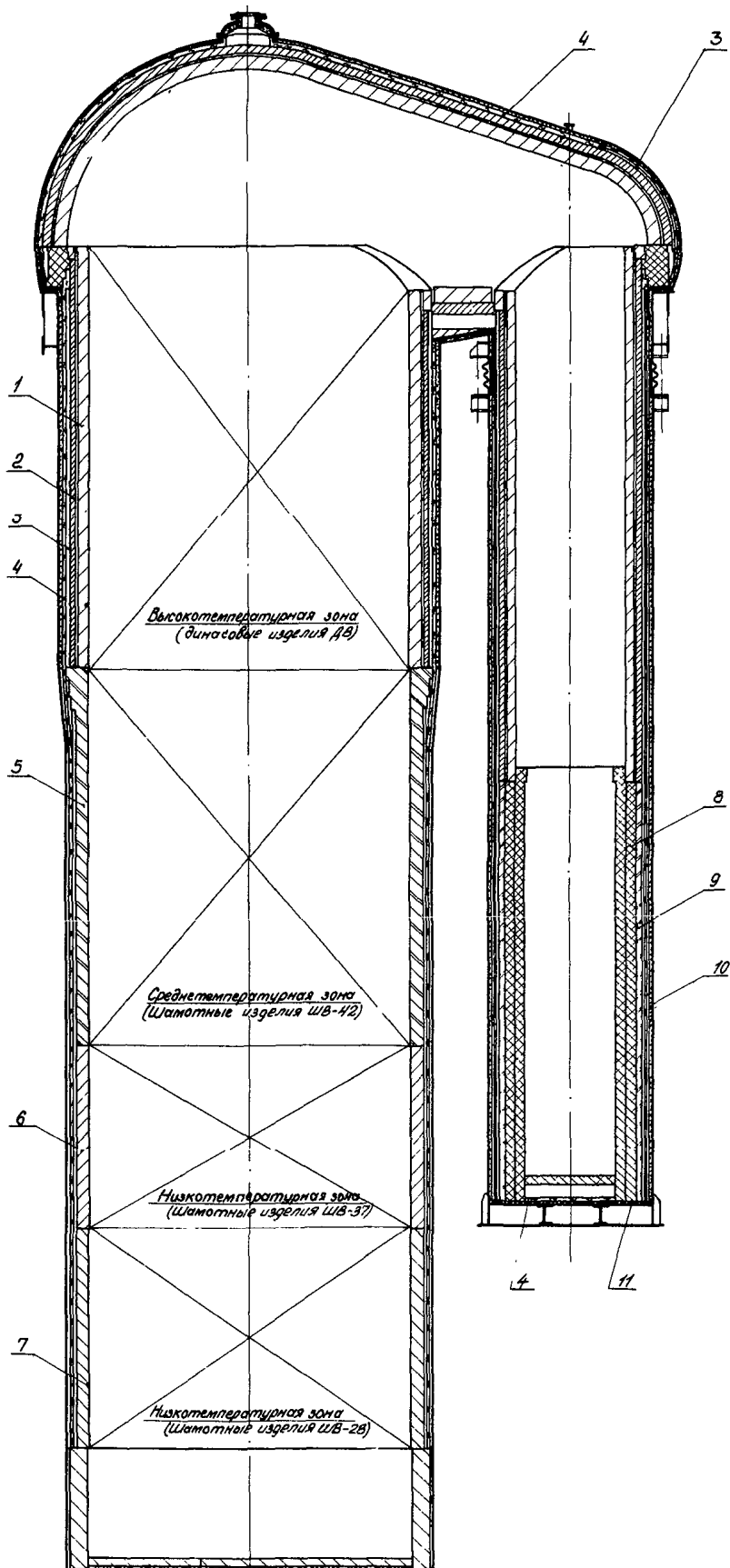
Рис. 35. Распределение огнеупоров в кладке воздухоподогревателя с выносной камерой горения и температурой под куполом до 1550°C.
