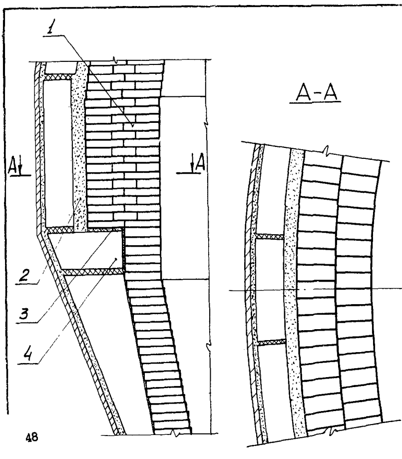
Рис.17. Кладка толстостенного распара пе- чи без мараторного кольца: 1 - шамотные каолиновые изделия; 2 - угле- родистая масса; 3 - шамотно-глинистая мас- са; 4 - горизонтальные холодильники
