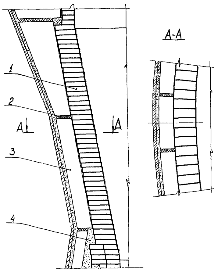
Рис.16. Кладка запечек: 1 - шамотные каолиновые изделия; 2 - чугу- нная замазка; 3 - периферийные плито- вые холодильники; 4 - углеродистая масса
