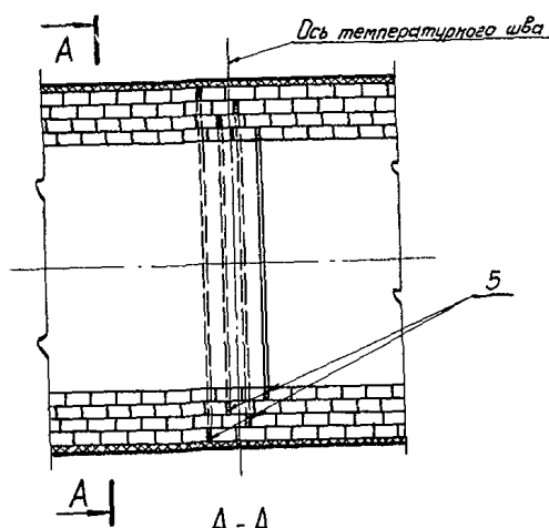
Рис.52. Кладка лаза в подкупольном пространстве 1 - высокоглиноземистые муллитокорундовые изделия;
