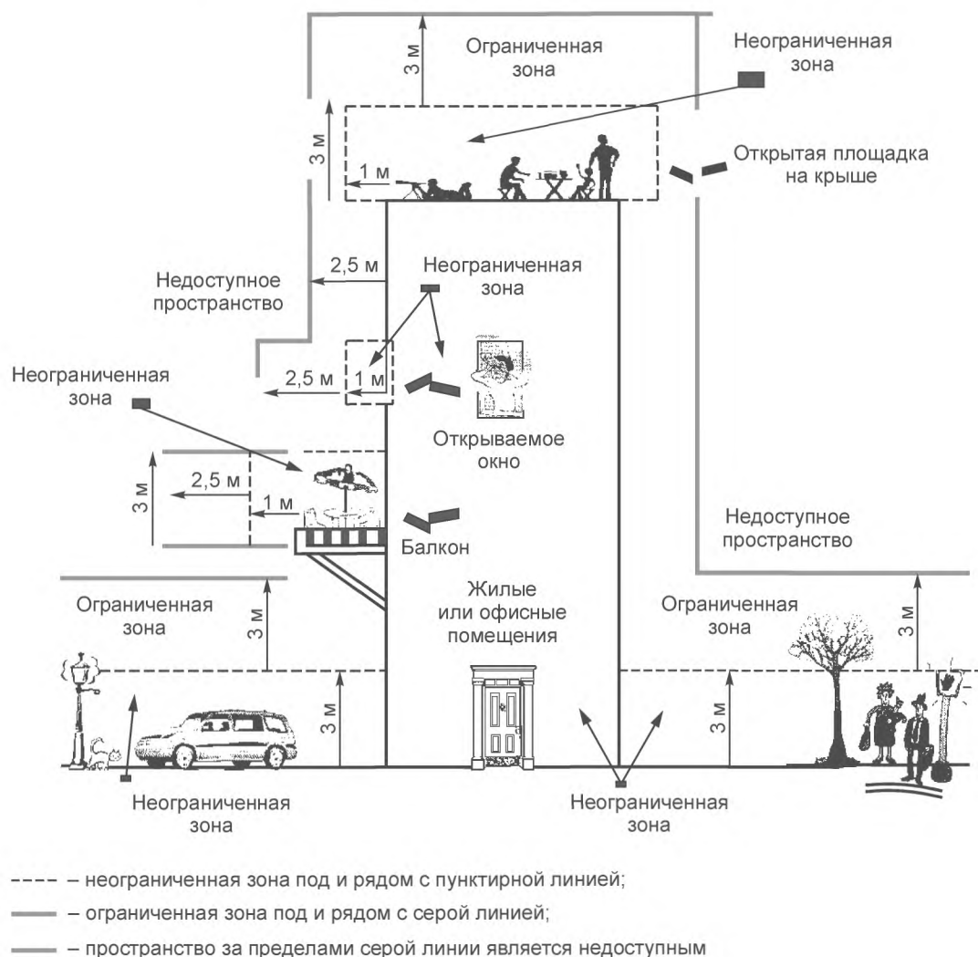
Рисунок 3 — Примеры вариантов внешнего расположения
