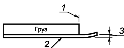
1 — нижний край магнитной полосы; 2 — испытуемая карта; 3 — загиб
