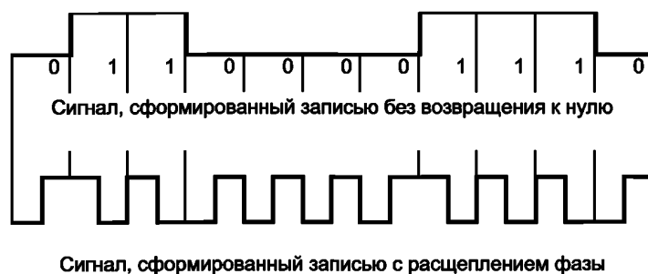
Рисунок В.2 — Кодирование с расщеплением фазы
