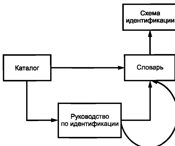
Рисунок 1 — Структура данных, определенная в комплексе стандартов ИСО 22745
