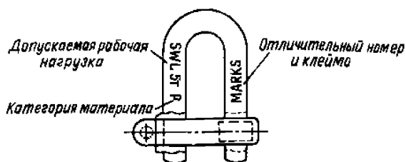
Рис. 11.2.1-3 Маркировка скобы
