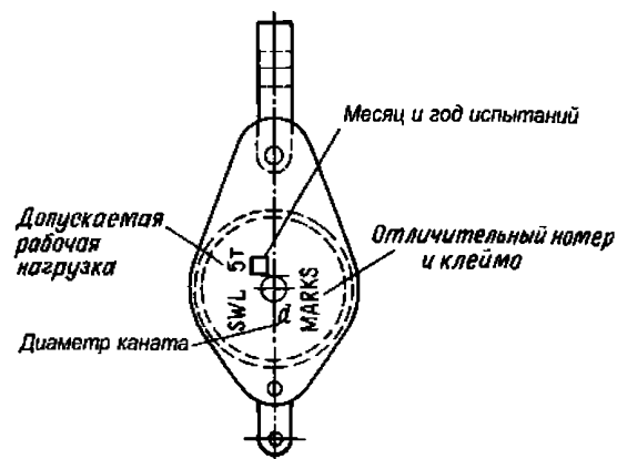
Рис. 11.2.1-5 Маркировка блока
