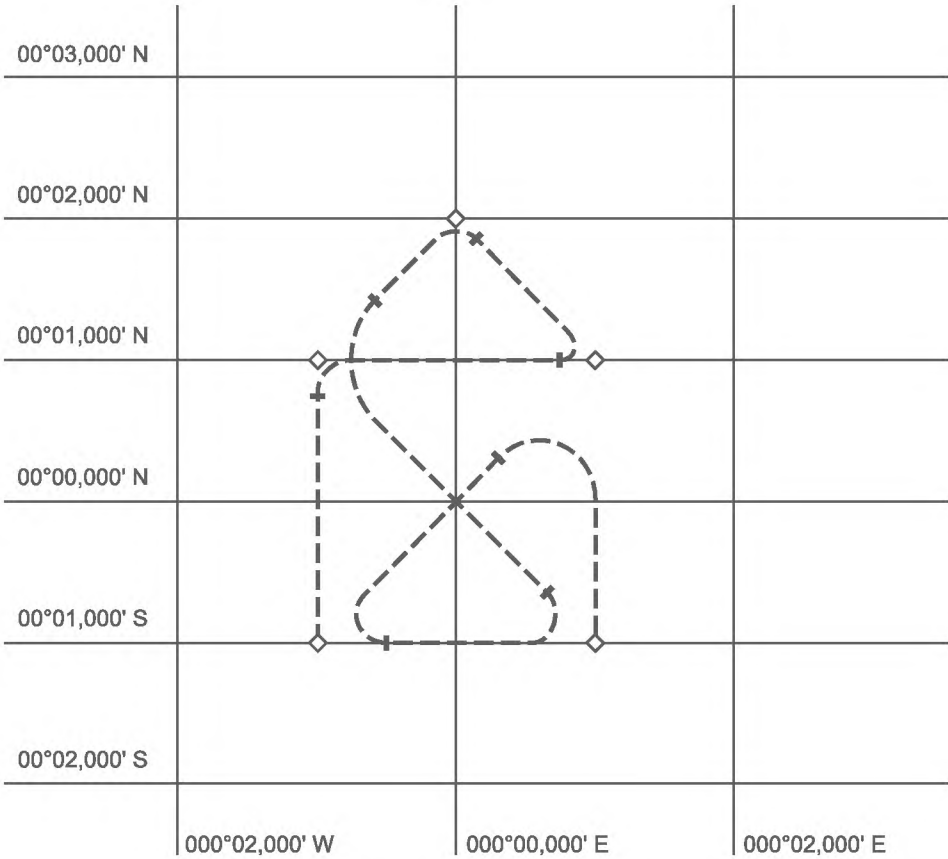
Рис. J.2 — Плавание по сценарию № 2
