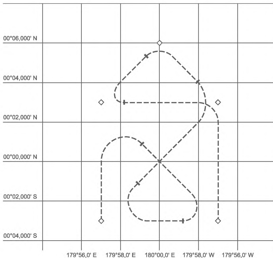
Рис. J.3 — Плавание по сценарию № 3
