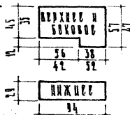
Сечения коробов
