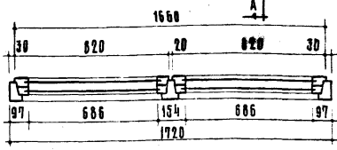
по Б-Б
