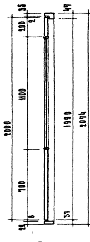
По а-а
