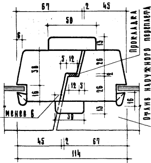
По 5-5
