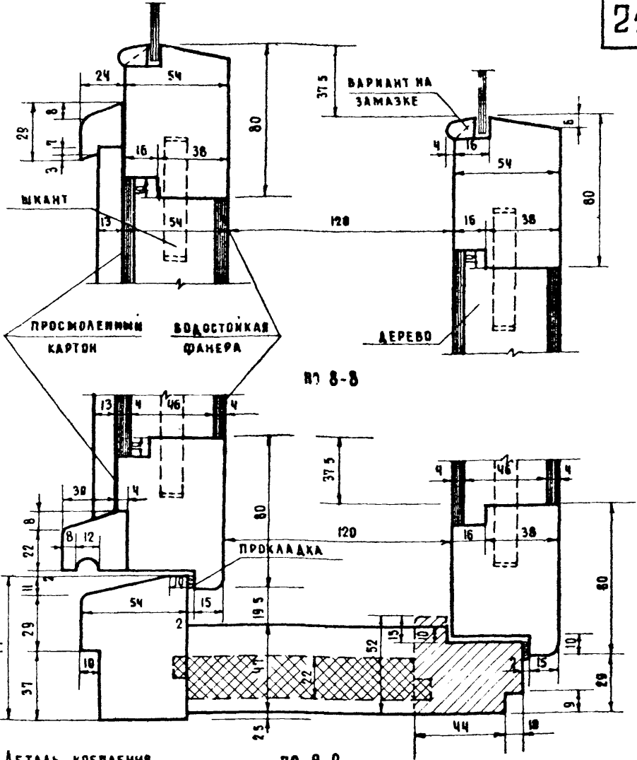
ДЕТАЛЬ КРЕПЛЕНИЯ U-ОБРАЗНОЙ ПРОКЛАДКИ. ГВОЗДИ Ф 8-10 ЧЕР 300-400 КЛЕЙ 88
