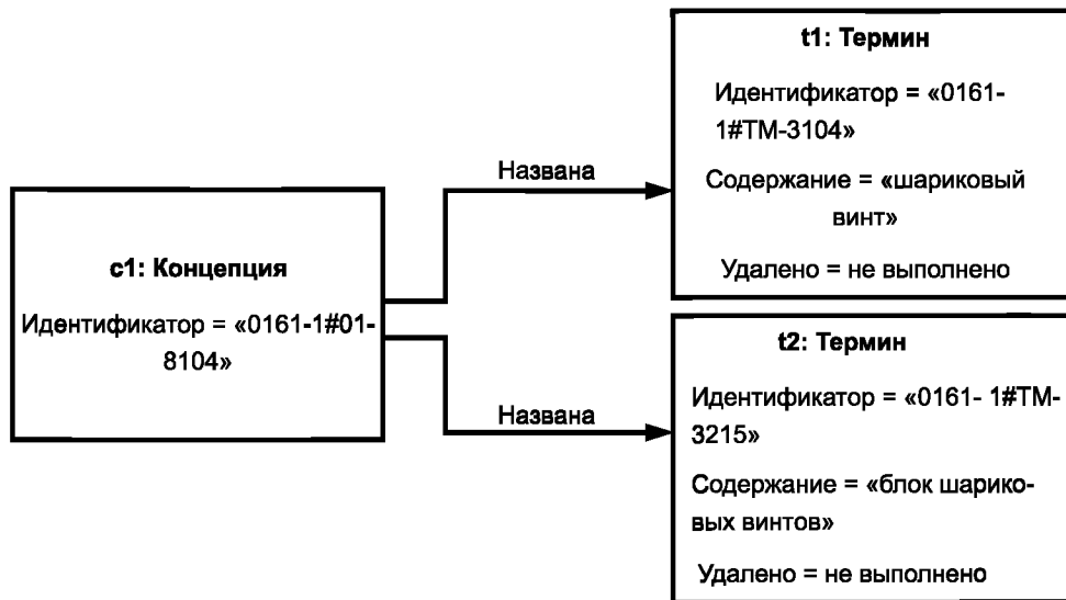
Рисунок D.2 — Состояние OTD после добавления неправильно написанного термина
