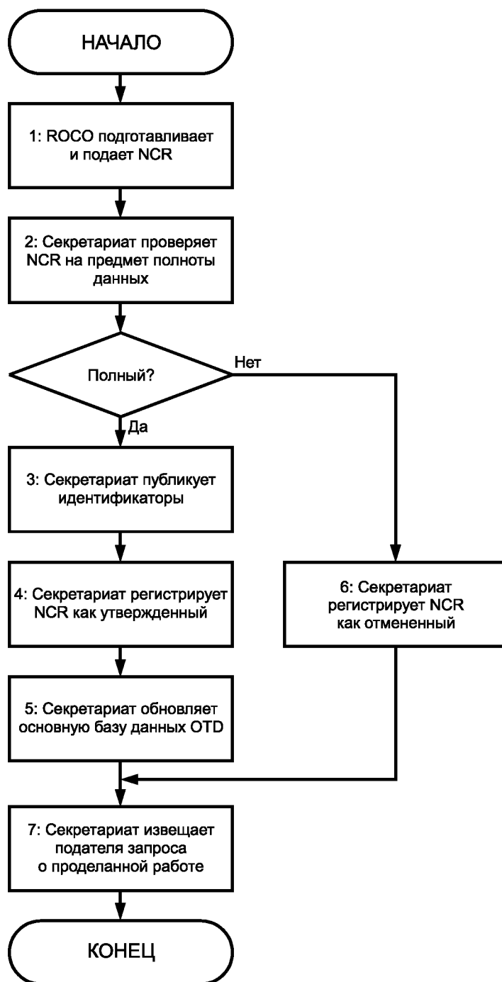
Рисунок 2 — Процедура добавления концепции
