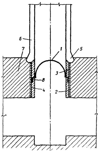
Рис. 6. Схема герметичной перемычки в нижней части ствола
