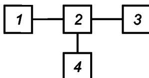
1 — измерительный генератор; 2 — коаксиальный соединитель; 3 — поверяемый вольтметр; 4 — эталонный частотомер
