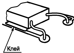
Рисунок А.4 — Боковой монтаж
