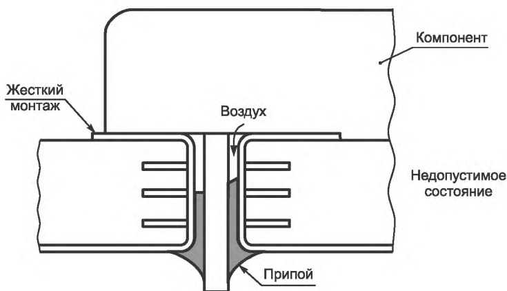
Рисунок 2 — Непропай отверстий
