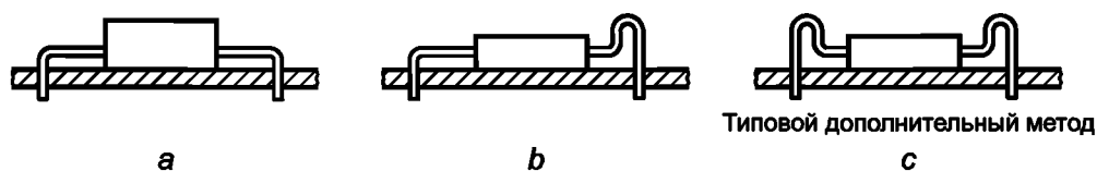
Рисунок А.8 — Примеры формы выводов
