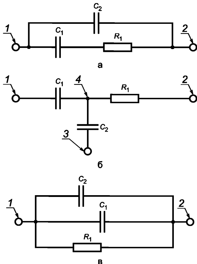
Рисунок В.3 — Составные меры тангенса угла потерь
