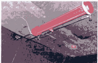
Рисунок Д6 – Состояние трубы D_{\text{наруж}} 125 \text{ мм} до и после испытаний (максимальная температура пожара 340–500 °С)
