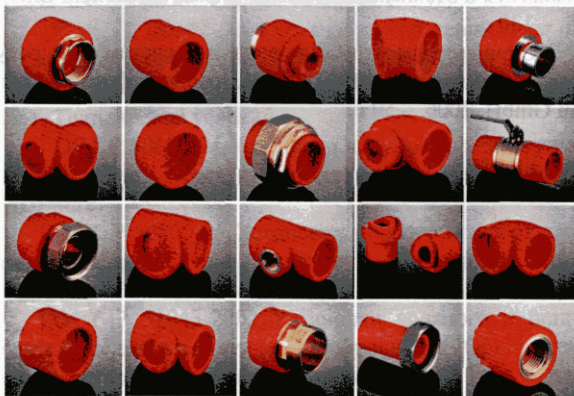
Рисунок А2 – Общий вид фитингов
