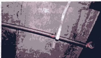
Рисунок Д5 – Состояние трубы D_{\text{наруж}} 32 \text{ мм} до и после испытаний (максимальная температура пожара 360–500 °С)
