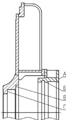
Карта дефектации и ремонта 2
