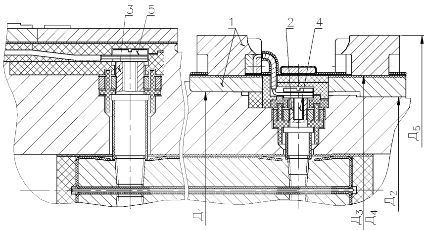
Рисунок 7.3 – Контактные кольца с токоподводом, поз.2 рис. 7.1а и 7.1б
