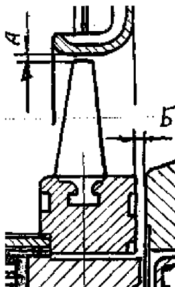
Рисунок 8.2 - Зазор между вентилятором и обтекателем
