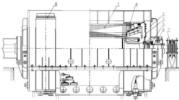
1 – статор; 2 – щит наружный; 3 – обтекатель; 4 – ротор; 5 – уплотнение вала ротора;
