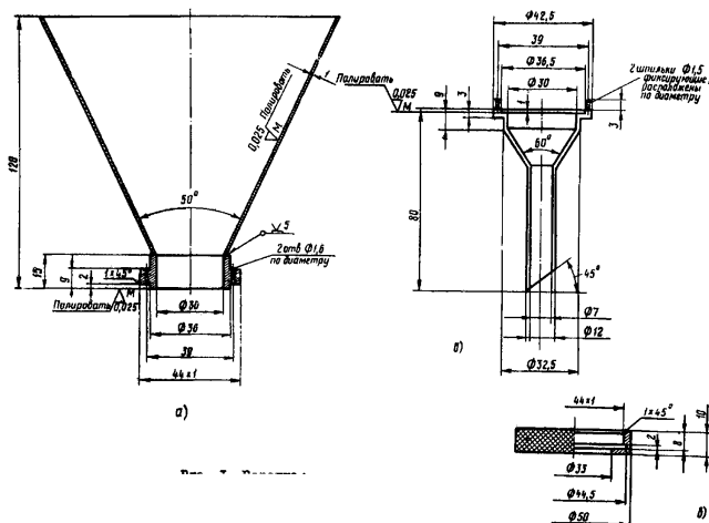
а – верхняя часть (вместимость 600 мл); б – нижняя часть; в – накидная гайка.
